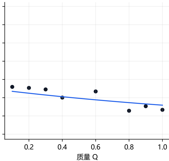
N=1B, D=150B
