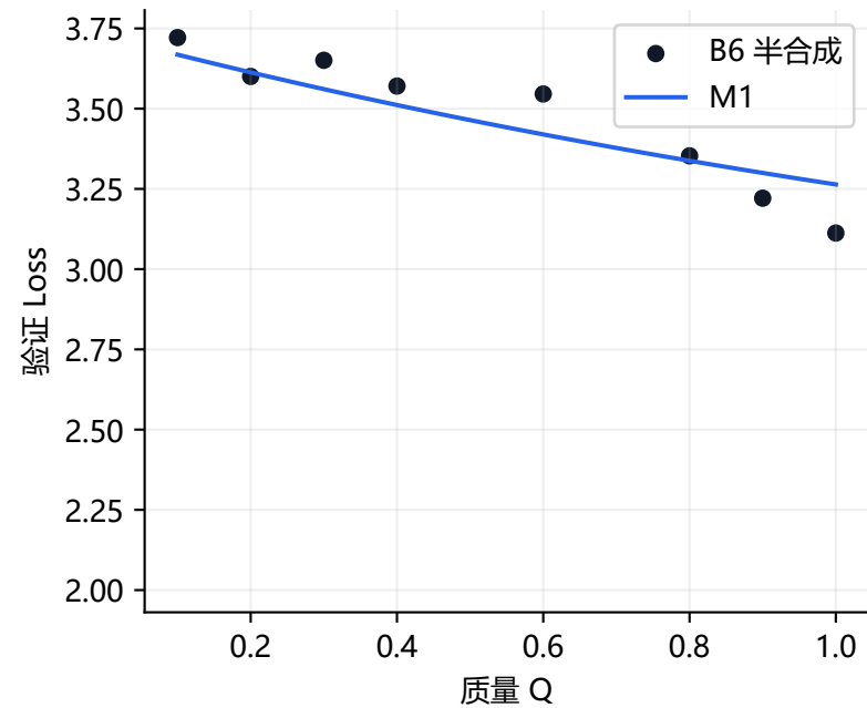
N=0.07B, D=10B
