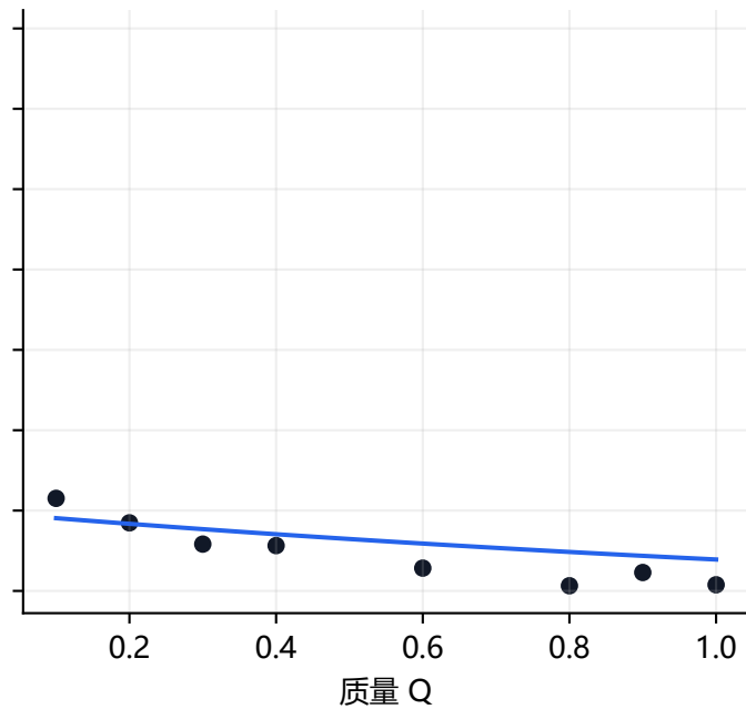
N=11.97B, D=600B
