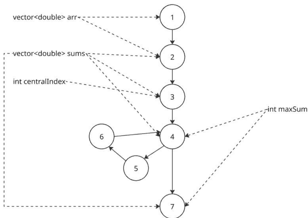
Информационный граф
