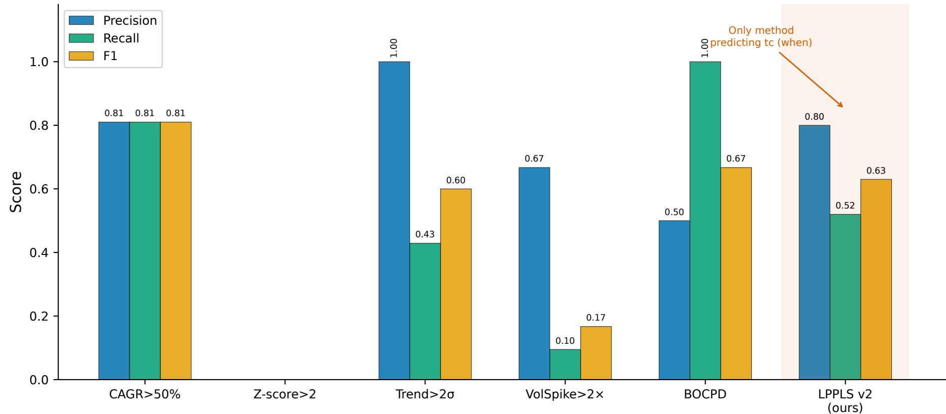
PhaseBreak v2 vs. Baselines — Precision / Recall / F1 (Finance domain, n=42)
