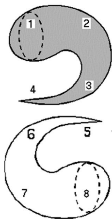
Рис. 4. Модель «А», полученная растяжением «инь-ян».
