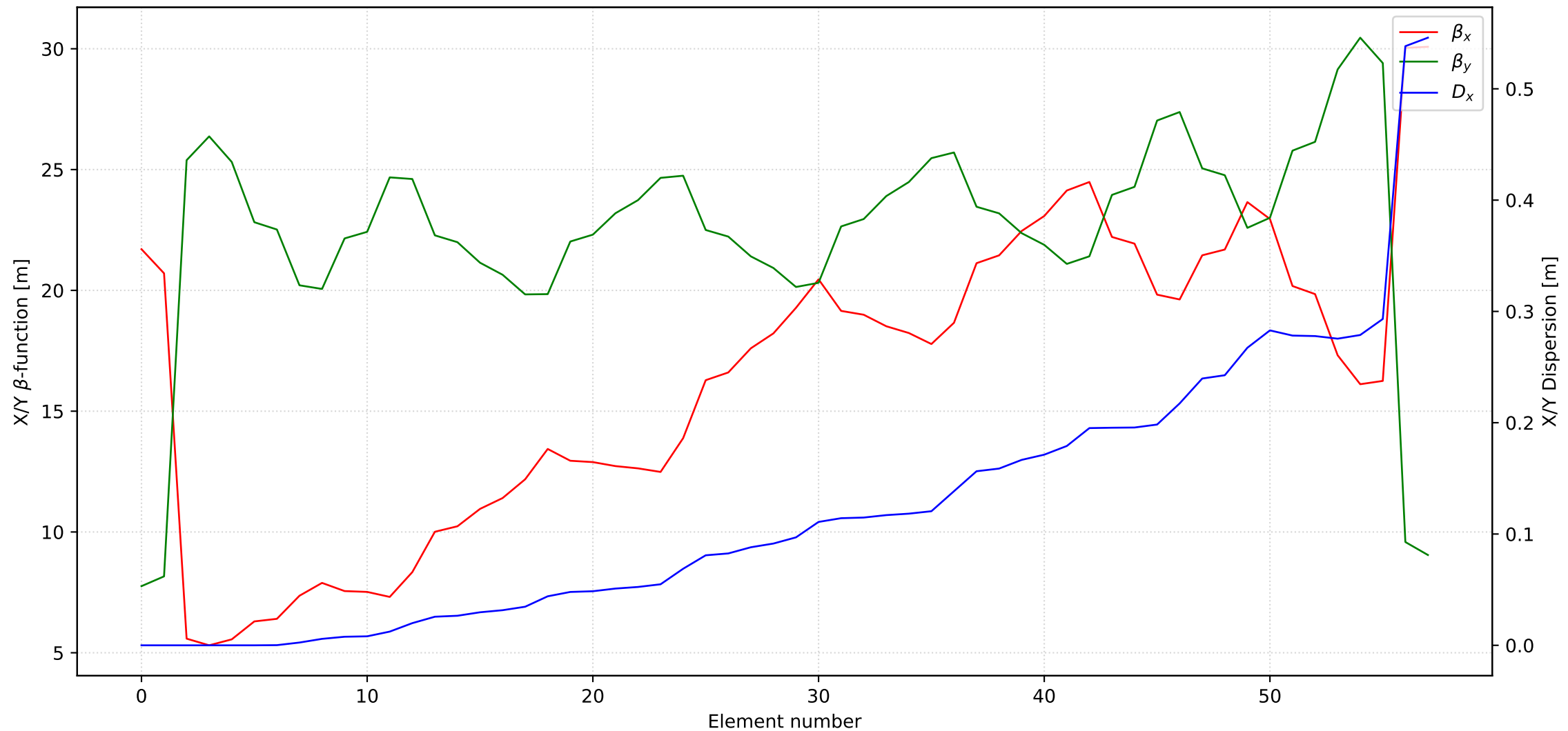
Twiss Parameters vs Element Number
