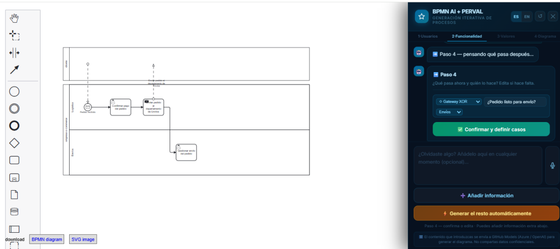
Figura 7.5: Generación paso a paso del flujo del proceso. El sistema propone una puerta exclusiva (XOR).
