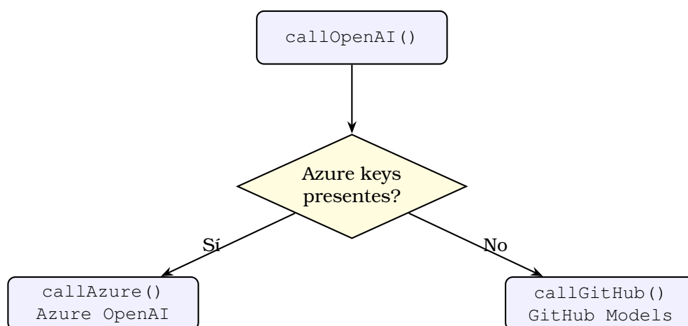
Figura B.1: Selección dinámica de proveedor LLM en llm.js . callOpenAI actúa como punto de entrada único e independiente del backend .
