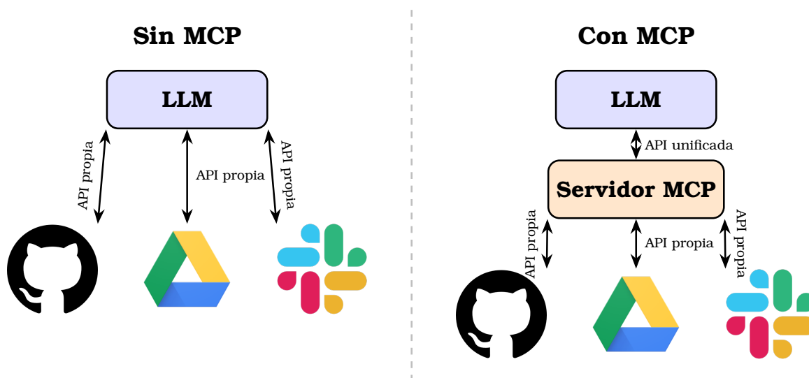
Figura 2.2: Comparación entre la integración directa del LLM con herramientas externas mediante APIs propias (izquierda) y la integración estandarizada a través del protocolo MCP (derecha).
