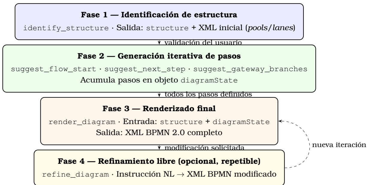
Figura 5.3: Fases del flujo de generación y refinamiento iterativo de modelos BPMN. La fase 4 puede ejecutarse tantas veces como el usuario lo requiera.
