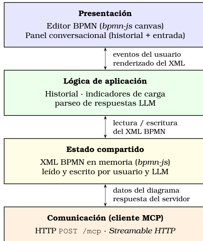
Figura 5.2: Estructura por capas de la extensión sobre bpmn.io.
