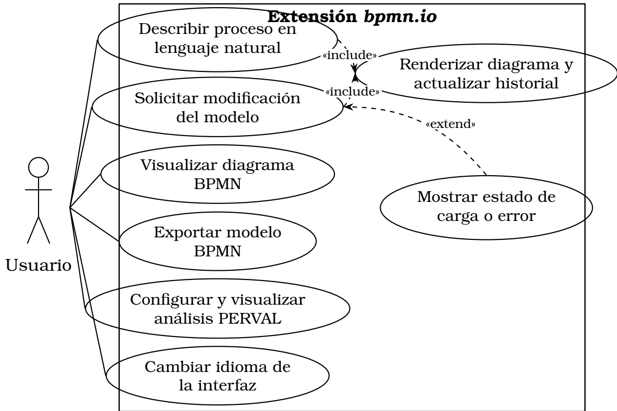
Figura 3.5: Diagrama de casos de uso de la extensión sobre bpmn.io.
