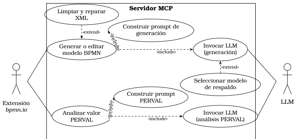
Figura 3.6: Diagrama de casos de uso del servidor MCP y del módulo de análisis PERVAL.
