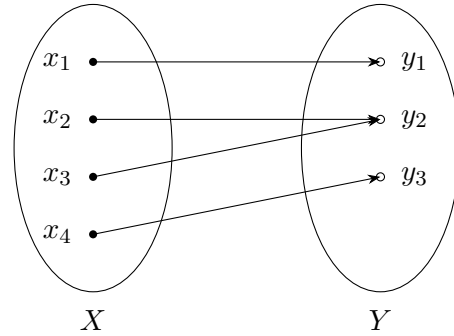
Aplicación sobreyectiva pero no inyectiva
