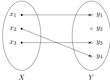
Aplicación inyectiva pero no sobreyectiva
