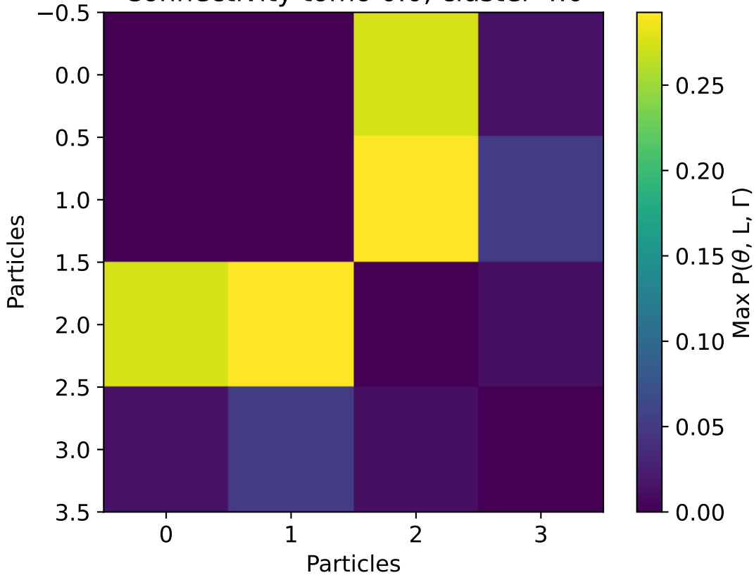
Connectivity tomo 0.0, cluster 4.0
