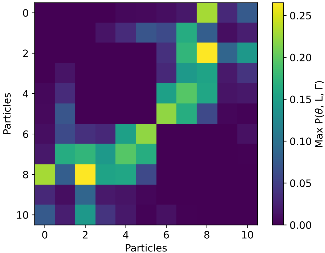
Connectivity tomo 0.0, cluster 11.0
