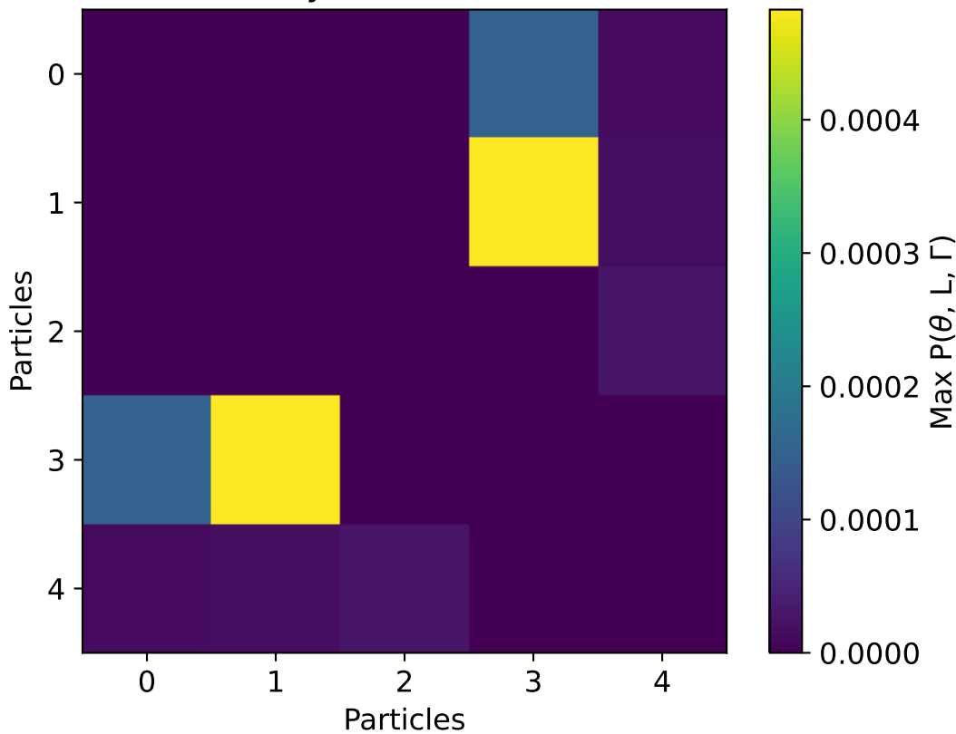
Connectivity tomo 0.0, cluster 5.0
