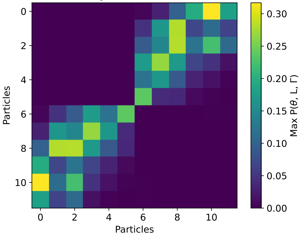
Connectivity tomo 0.0, cluster 12.0
