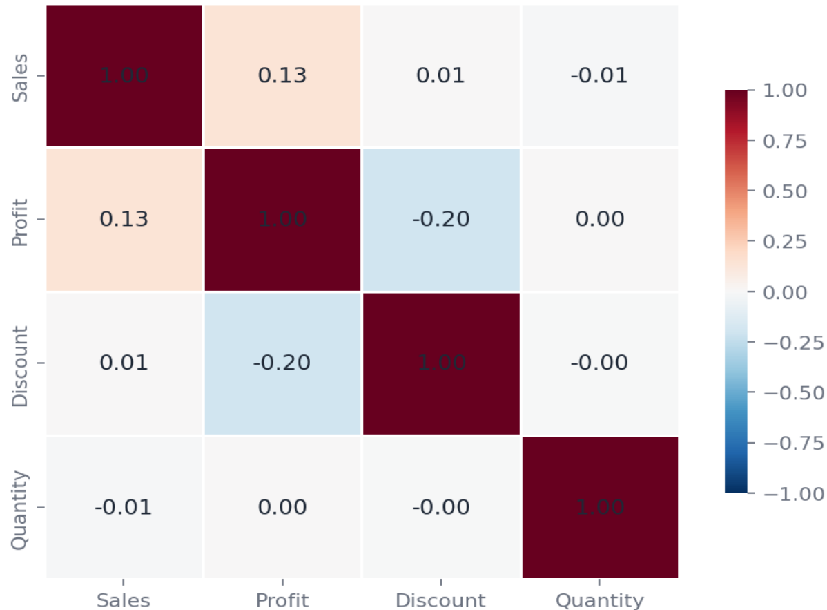
Matriz de correlación — paleta divergente, centrada en 0
