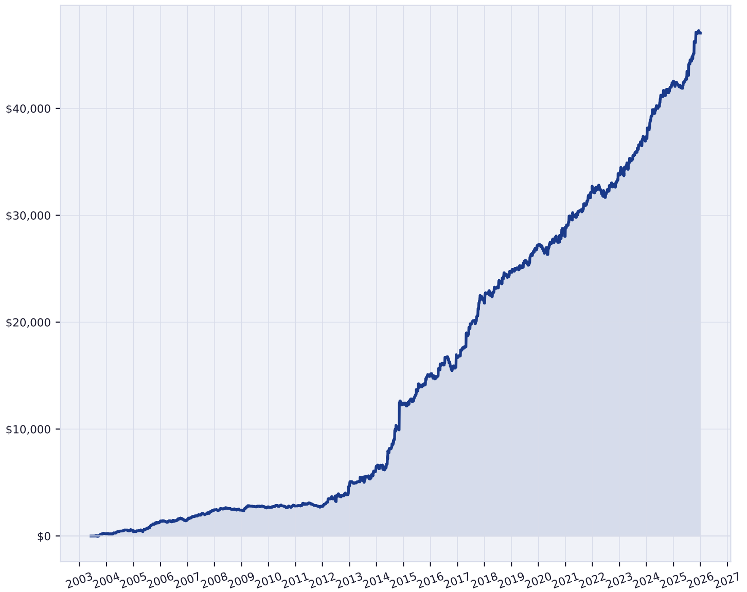
Cumulative P&amp;L
