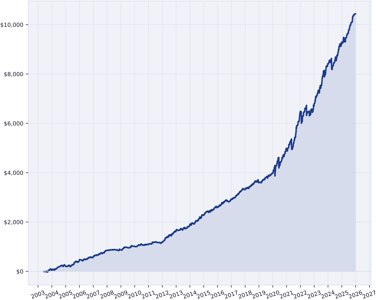
Cumulative P&L
