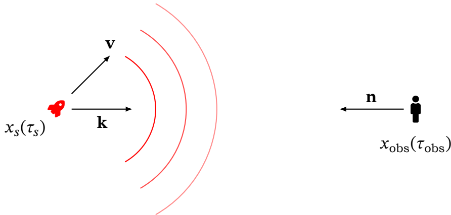
Рис. 7.1. Геометрія ефекту Доплера: \mathbf{k} — хвильовий вектор, \mathbf{n} — одиничний вектор від спостерігача до джерела.
