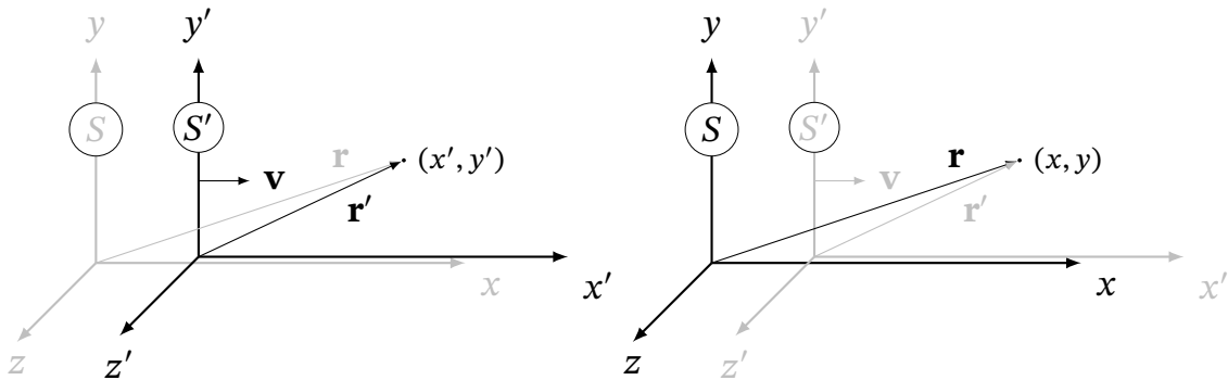
Рис. 5.1. Дві інерціальні системи відліку S й S' , де S' рухається вздовж осі x зі швидкістю v відносно S . Показано радіус-вектори події \mathbf{r} і \mathbf{r}' та відповідні координати (x, y, z) і (x', y', z') . На рисунку для зручності показані осі OY та OY' .
