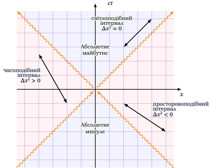
Рис. 5.2. Конус світла у просторі-часі Мінковського. Часоподібні інтервали між подіями ( \Delta s^2 > 0 ) мають нахил, менший за 45^\circ відносно осі ct , просторовоподібні ( \Delta s^2 < 0 ) — більший за 45^\circ , світлоподібні ( \Delta s^2 = 0 ) — рівно 45^\circ .
