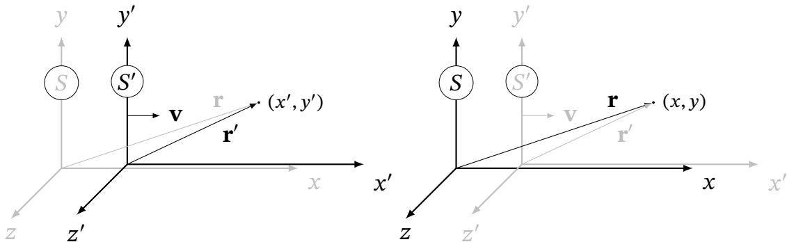
Рис. 5.1. Дві інерціальні системи відліку S і S' , де S' рухається вздовж осі x зі швидкістю v відносно S . Показано радіус-вектори події \mathbf{r} і \mathbf{r}' та відповідні координати (x, y, z) і (x', y', z') . На рисунку для зручності показані осі OY та OY' .
