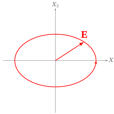
Рис. 3.5. Еліптична поляризація.
