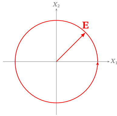
Рис. 3.3. Колова поляризація (випадок E_2 = iE_1 , обертання вектора E проти годинникової стрілки).
