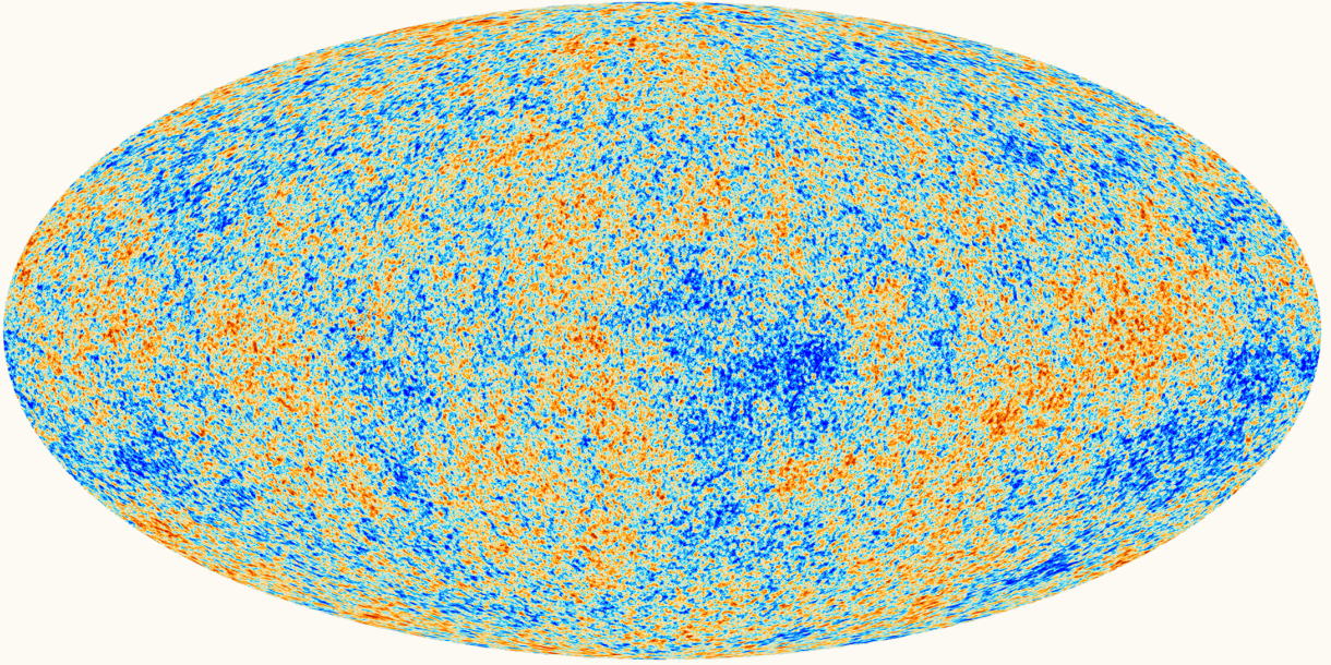
Рис. 7.1: Карта температурних анізотропій СМВ від місії Planck 2018 [3]. Кольори відображають відхилення від середнього T_0 = 2.725 \text{ K} у діапазоні \pm 300 \mu\text{K} — спостережуваний відбиток первинних флуктуацій інфлатона після \sim 380\,000 років еволюції. Зображення: ESA and the Planck Collaboration [31].
