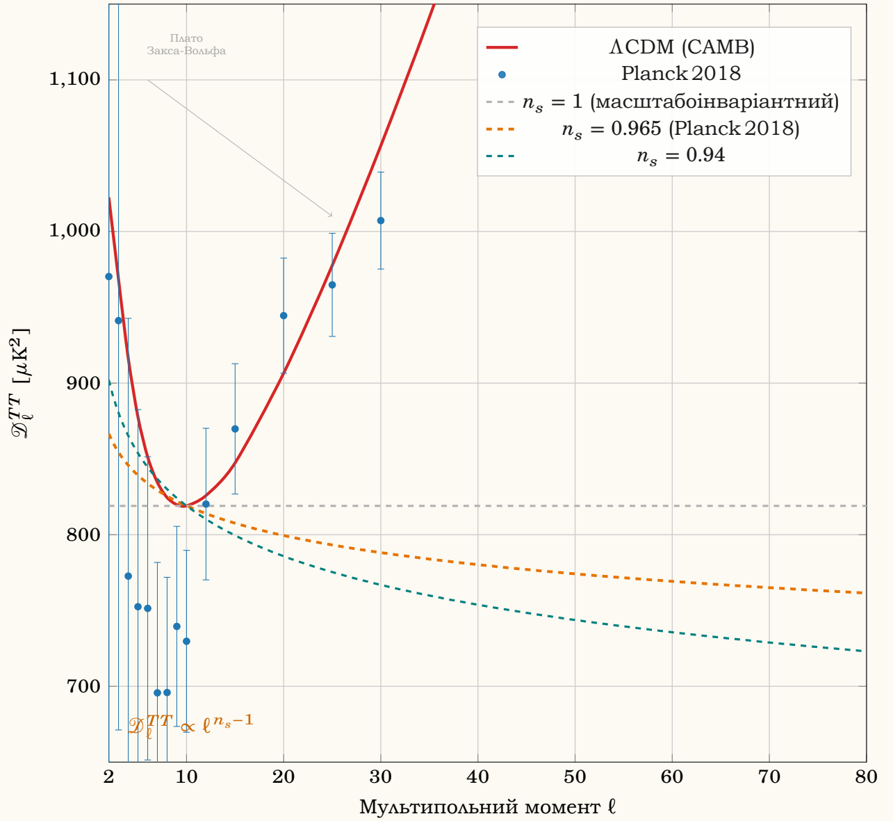
Рис. 7.3: Збільшений вигляд плато Закса–Вольфа ( 2 \leq \ell \lesssim 80 ) кутового спектра потужності \mathcal{D}_\ell^{TT} за даними місії Planck 2018 [3]. Штрихові лінії ілюструють нахил первинного спектра \mathcal{D}_\ell^{TT} \propto \ell^{n_s-1} для трьох значень спектрального індексу n_s . Горизонтальна лінія відповідає масштабоінваріантному спектру Гарісона–Зельдовича ( n_s = 1 ); відхилення від неї для планківського значення n_s = 0.965 \pm 0.004 підтверджує червоний нахил первинних скалярних збурень — базове передбачення інфляційних моделей повільного кочення поля. Усі криві нормовано в точці \ell = 10 , де \mathcal{D}_{10}^{\Lambda\text{CDM}} \approx 819 \mu K^2 .
