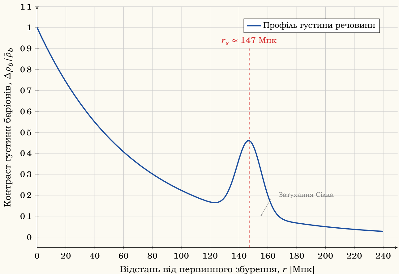
Рис. 6.3: Схематичний профіль поширення первинного адіабатичного збурення у баріонній компоненті плазми (модельна крива). Надлишок речовини на радіусі звукового горизонту r_s відповідає сучасному масштабу ВАО.
