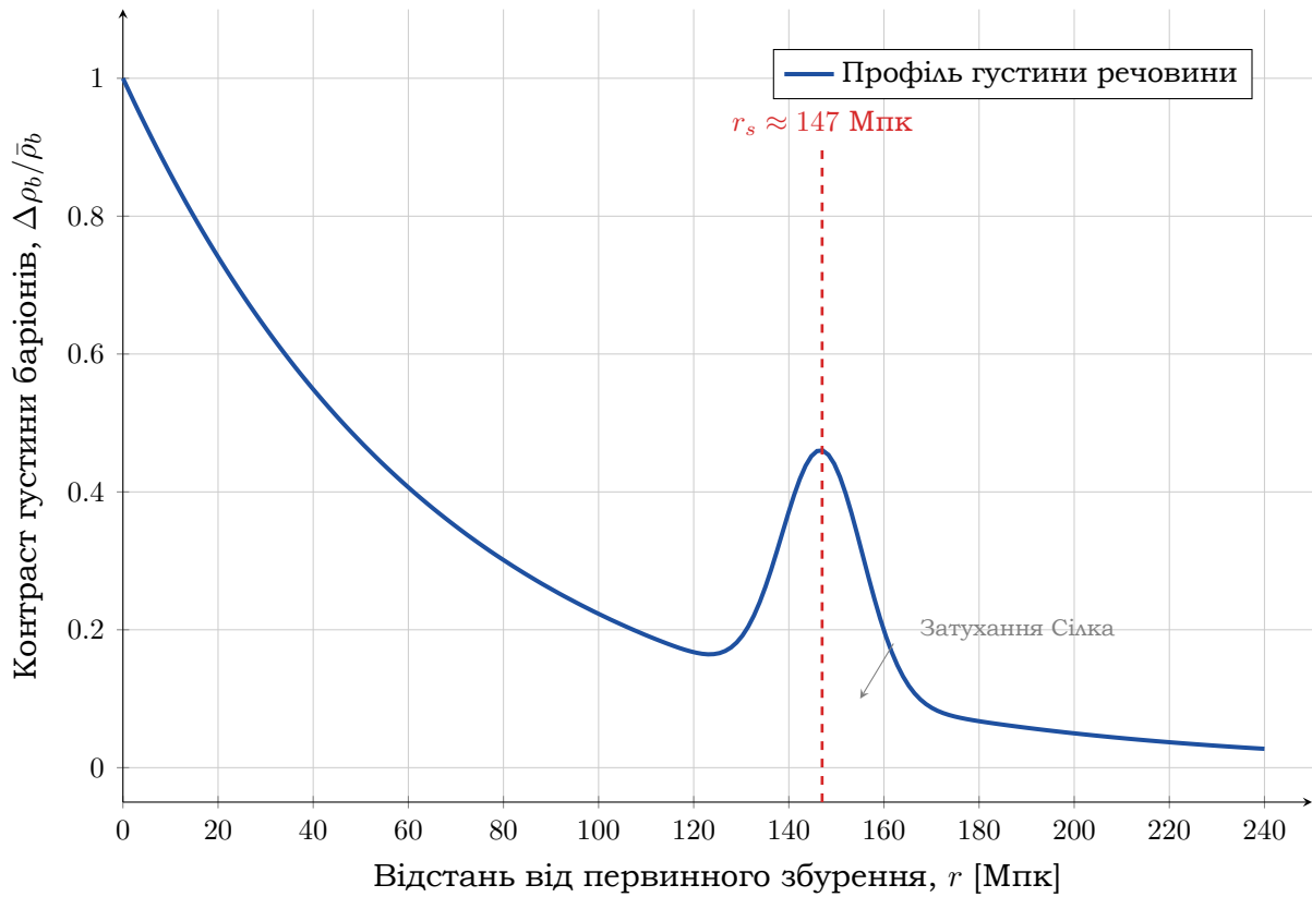
Рис. 6.3: Схематичний профіль поширення первинного адіабатичного збурення у баріонній компоненті плазми (модельна крива). Надлишок речовини на радіусі звукового горизонту r_s відповідає сучасному масштабу ВАО.
