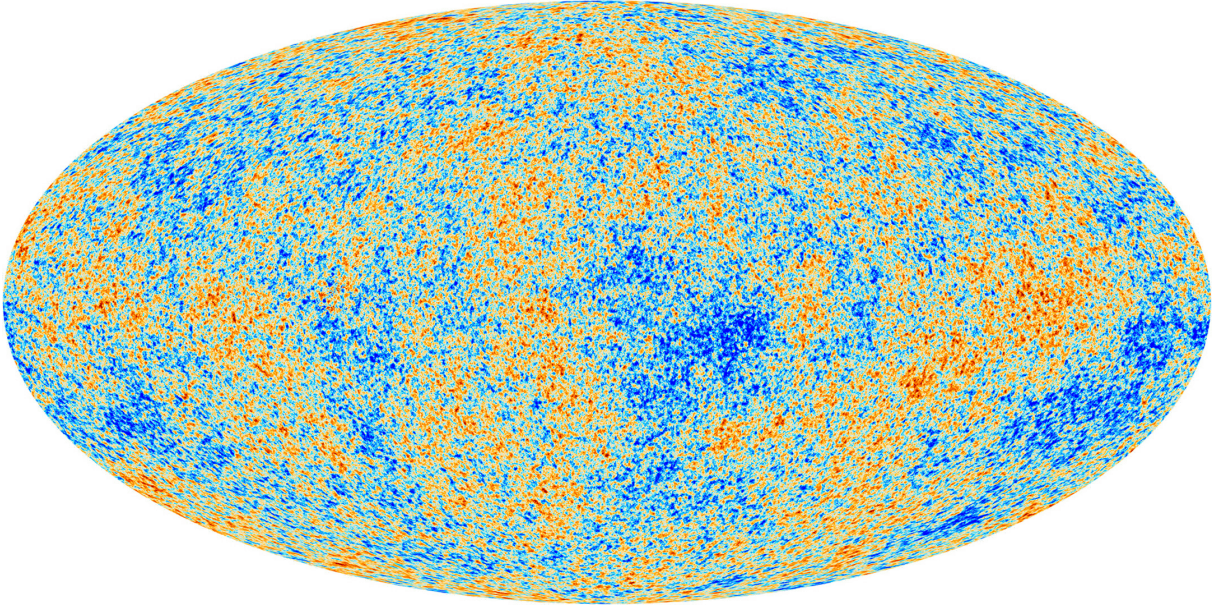
Рис. 7.1: Карта температурних анізотропій СМВ від місії Planck 2018 [1]. Кольори відображають відхилення від середнього T_0 = 2.725 К у діапазоні \pm 300 \mu\text{K} — спостережуваний відбиток первинних флуктуацій інфлатона після \sim 380\,000 років еволюції. Зображення: ESA and the Planck Collaboration [32].
