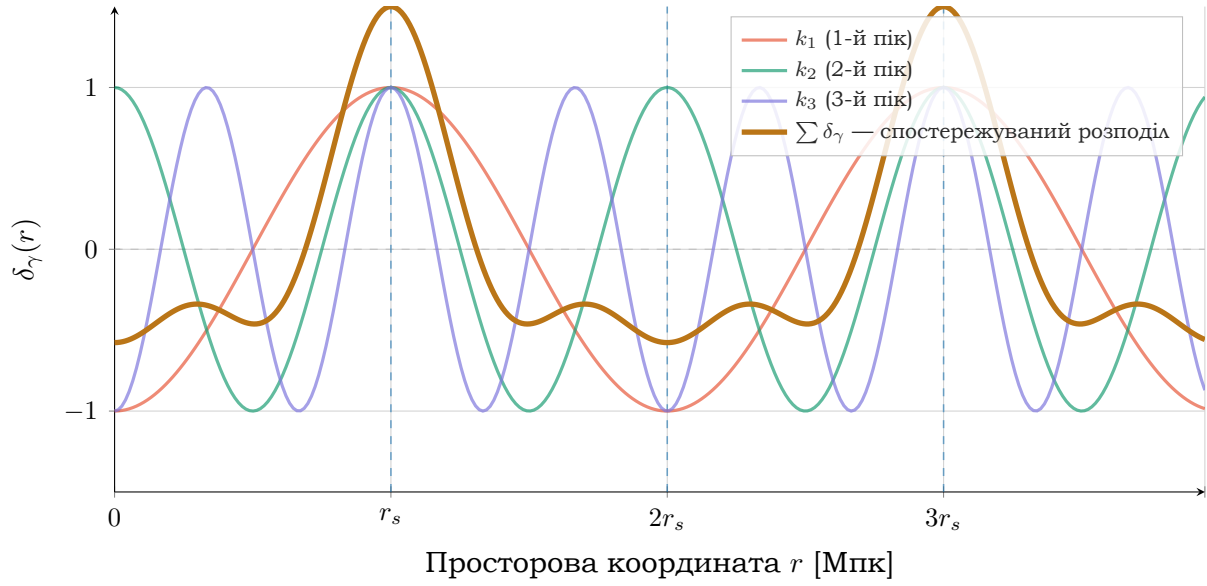
Рис. 6.1: Просторовий «знімок» розподілу \delta_\gamma(r) у момент рекомбінації — суперпозиція мод, заморожених у різних амплітудах (пор. з рис. 6.2). Бурштинова крива — спостережуваний сигнал, що кодується у кутовий спектр \mathcal{D}_\ell^{TT} . Пунктирні вертикалі — масштаби r_s, 2r_s, 3r_s \approx 147 Мпк, що відповідають акустичним пікам.
