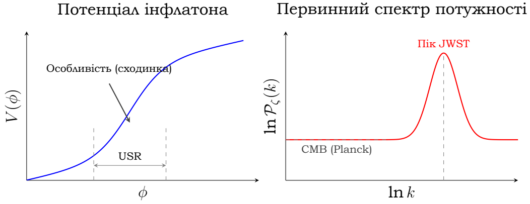
Рис. 9.1: Схематичне зображення механізму генерації зламаного спектра. Ліворуч: потенціал інфлатона з короткою ділянкою ультра-повільного кочення (USR — ultra-slow roll), де класична швидкість поля падає. Праворуч: відповідний спектр потужності кривини \mathcal{P}_\zeta(k) , що зберігає масштабну інваріантність на масштабах CMB, але має локальний надлишок амплітуди на високих хвильових числах.
