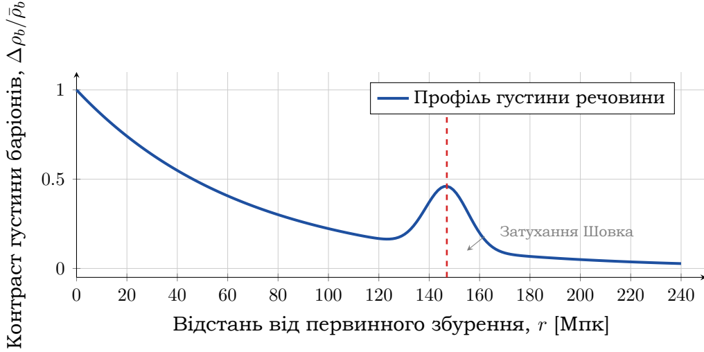
Рис. 1: Профіль поширення первинного адіабатичного збурення у баріонній компоненті плазми. Чітко виражений надлишок речовини на радіусі звукового горизонту r_s відповідає сучасному масштабу ВАО.
