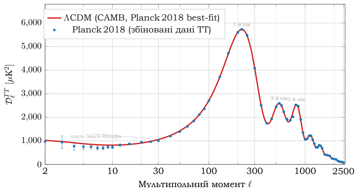
Рис. 2: Кутовий ТТ-спектр потужності СМВ. Точки — дані Planck 2018 [planck2018params]. Крива — базова модель \Lambda CDM, розрахована CAMB з параметрами таблиці ???. Видно три акустичні піки та плато Закса-Вольфа на великих кутових масштабах ( \ell \lesssim 30 ).
