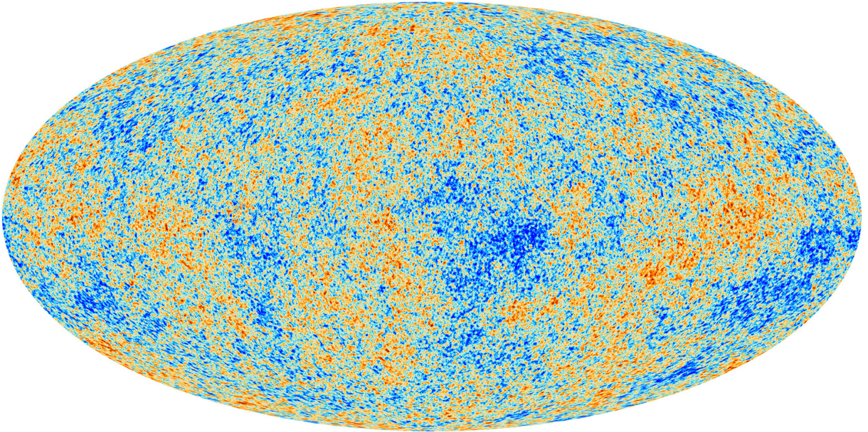
Рис. 3: Карта температурних анізотропій СМВ від місії Planck 2018 [1]. Кольори відображають відхилення від середнього T_0 = 2.725 \text{ K} у діапазоні \pm 300 \mu\text{K} — спостережуваний відбиток первинних флуктуацій інфлатона після \sim 380\,000 років еволюції. Зображення: ESA and the Planck Collaboration [20].
