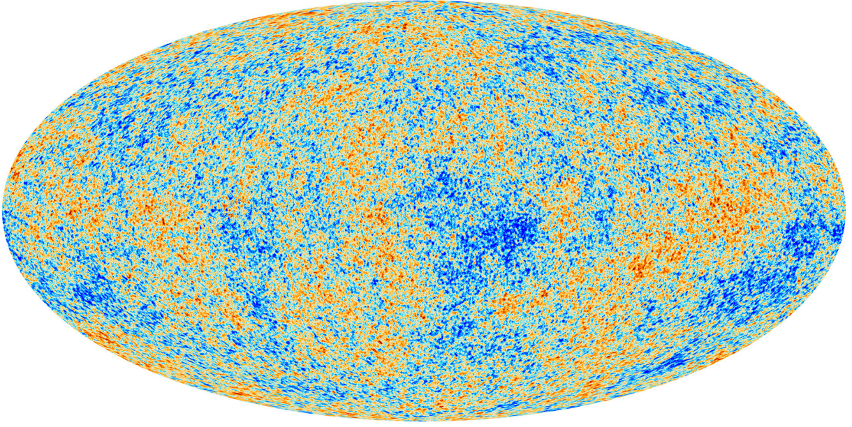
Рис. 7.1: Карта температурних анізотропій СМВ від місії Planck 2018 [1]. Кольори відображають відхилення від середнього T_0 = 2.725 \text{ K} у діапазоні \pm 300 \mu\text{K} — спостережуваний відбиток первинних флуктуацій інфлатона після \sim 380\,000 років еволюції. Зображення: ESA and the Planck Collaboration [24].
