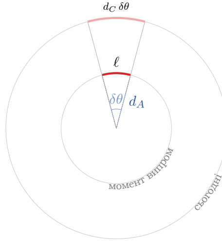
Рис. 1.1: Кутова відстань d_A = \ell/\delta\theta . Об'єкт фізичного розміру \ell видно під кутом \delta\theta ; через розширення d_A = d_C/(1+z) < d_C .
