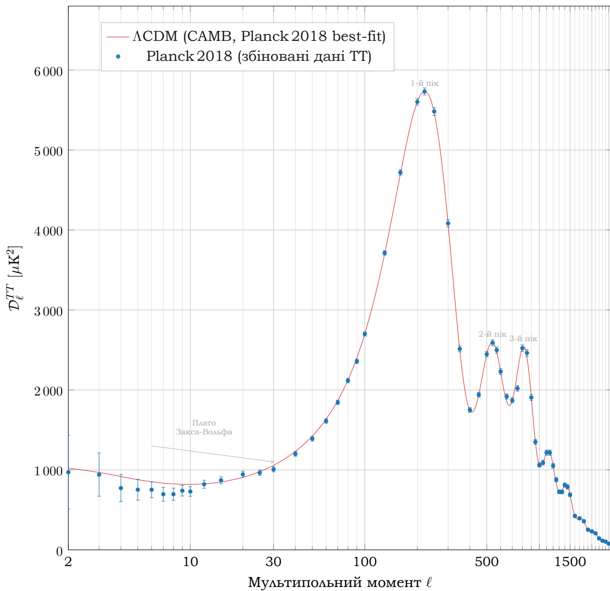
Рис. 7.2: Кутовий спектр потужності температурної анізотропії реліктового випромінювання за даними космічної місії Planck 2018 . Суцільна червона лінія відповідає найкращому фіту стандартної космологічної моделі \Lambda CDM.
