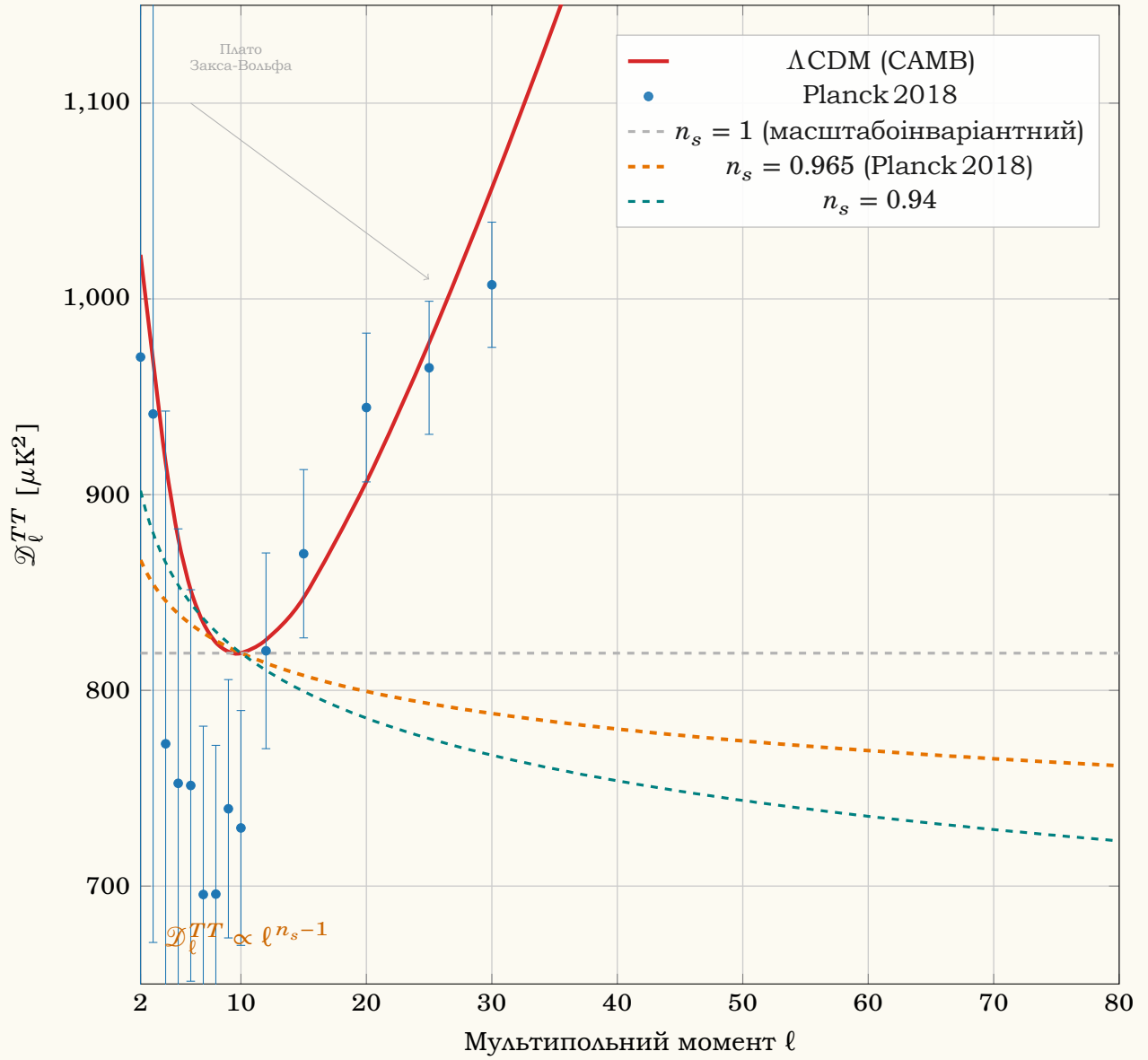
Рис. 7.3: Збільшений вигляд плато Закса–Вольфа ( 2 \leq \ell \lesssim 80 ) кутового спектра потужності \mathcal{D}_\ell^{TT} за даними місії Planck 2018 [1]. Штрихові лінії ілюструють нахил первинного спектра \mathcal{D}_\ell^{TT} \propto \ell^{n_s-1} для трьох значень спектрального індексу n_s . Горизонтальна лінія відповідає масштабоінваріантному спектру Гарісона–Зельдовича ( n_s = 1 ); відхилення від неї для планківського значення n_s = 0.965 \pm 0.004 підтверджує червоний нахил первинних скалярних збурень — базове передбачення інфляційних моделей повільного кочення поля. Усі криві нормовано в точці \ell = 10 , де \mathcal{D}_{10}^{\Lambda\text{CDM}} \approx 819 \mu K^2 .
