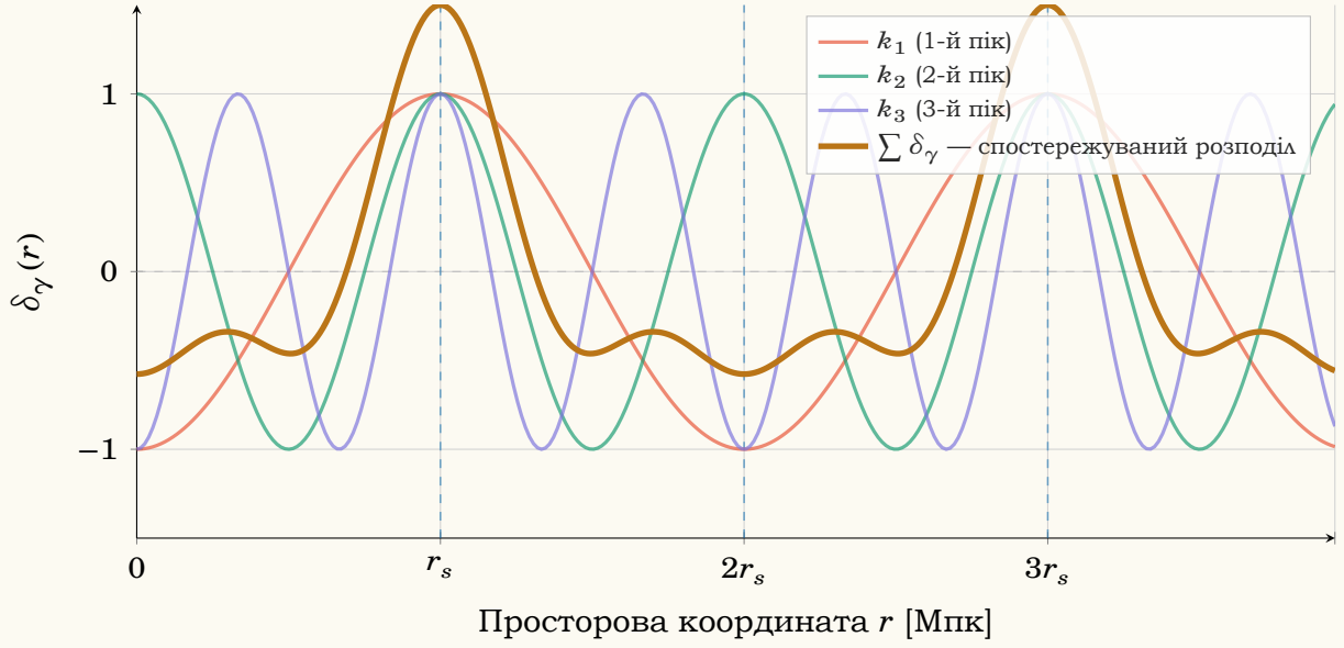
Рис. 6.1: Просторовий «знімок» розподілу \delta_\gamma(r) у момент рекомбінації — суперпозиція мод, заморожених у різних амплітудах (пор. з рис. 6.2). Бурштинова крива — спостережуваний сигнал, що кодується у кутовий спектр \mathcal{D}_\ell^{TT} . Пунктирні вертикалі — масштаби r_s , 2r_s , 3r_s \approx 147 Мпк, що відповідають акустичним пікам.
