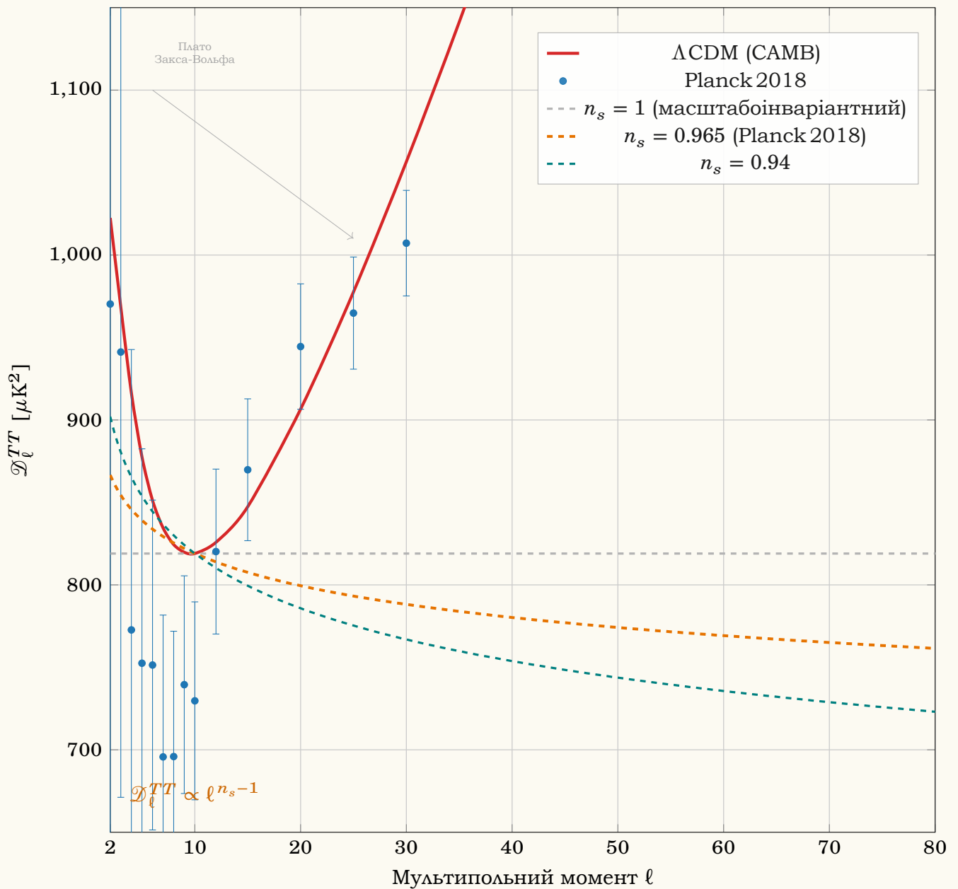
Рис. 7.3: Збільшений вигляд плато Закса-Вольфа ( 2 \leq \ell \leq 80 ) кутового спектра потужності \mathcal{D}_\ell^{TT} за даними місії Planck 2018 [3]. Штрихові лінії ілюструють нахил первинного спектра \mathcal{D}_\ell^{TT} \propto \ell^{n_s-1} для трьох значень спектрального індексу n_s . Горизонтальна лінія відповідає масштабоінваріантному спектру Гарісона-Зельдовича ( n_s = 1 ); відхилення від неї для планківського значення n_s = 0.965 \pm 0.004 підтверджує червоний нахил первинних скалярних збурень — базове передбачення інфляційних моделей повільного кочення поля. Усі криві нормовано в точці \ell = 10 , де \mathcal{D}_{10}^{\Lambda\text{CDM}} \approx 819 \mu\text{K}^2 .
