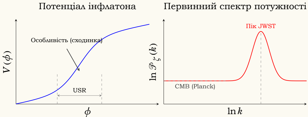
Рис. 2.2: Схематичне зображення механізму генерації зламаного спектра. Ліворуч: потенціал інфлатона з короткою ділянкою ультра-повільного кочення (USR — ultra-slow roll), де класична швидкість поля падає. Праворуч: відповідний спектр потужності кривини \mathcal{P}_\zeta(k) , що зберігає масштабну інваріантність на масштабах CMB, але має локальний надлишок амплітуди на високих хвильових числах.
