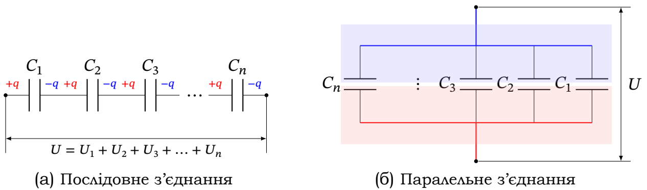
Рис. 6.3. З'єднання конденсаторів: (а) послідовне — заряд на всіх обкладках однаковий, напруги додаються; (б) паралельне — напруга на всіх конденсаторах однакова, заряди додаються
