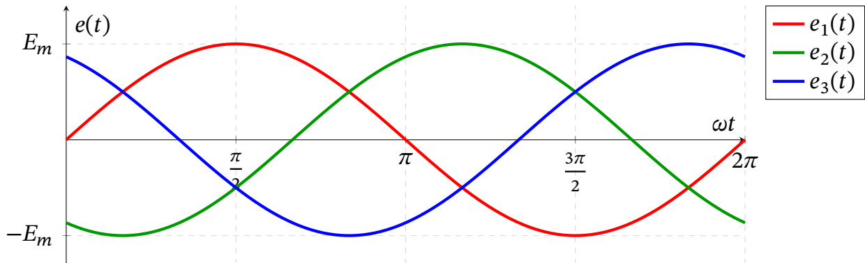
Рис. 17.20. Часові діаграми симетричної трифазної системи ЕРС
