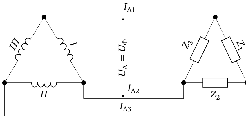
Рис. 17.23. Схема з'єднання генератора та приймача трикутником
