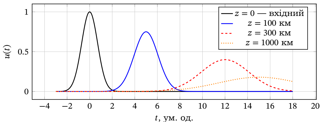
Рис. 18.3. Дисперсійне спотворення гаусового імпульсу при поширенні в лінії з втратами. З відстанню імпульс розширюється і зменшується за амплітудою — саме ця проблема мучила перші трансатлантичні кабелі.
