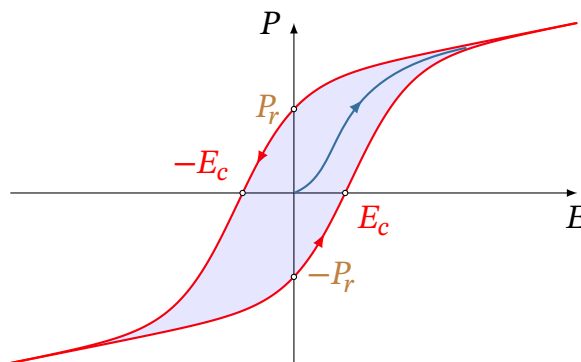
Рис. 5.14. Петля гістерезису сегнетоелектрика: P_r — залишкова поляризація, E_c — коерцитивна сила
