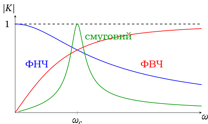
Рис. 17.18. Амплітудно-частотні характеристики трьох фільтрів: ФНЧ (синій), ФВЧ (червоний) і смугового (зелений). Для смугового прийнято Q = 5 .
