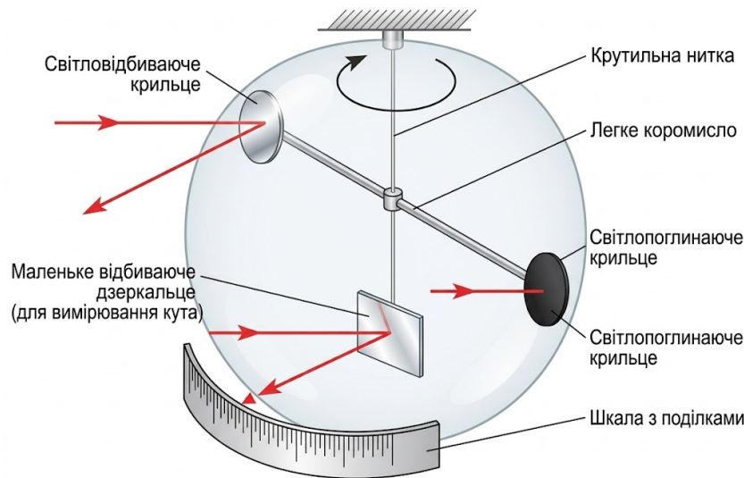
Рис. 15.6. Схема досліду П. М. Лебедєва (1899 р.) з вимірювання тиску світла
