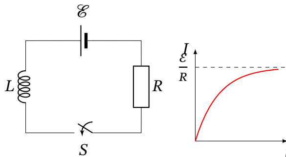
Рис. 11.11. Встановлення струму в колі з індуктивністю після замикання ключа
