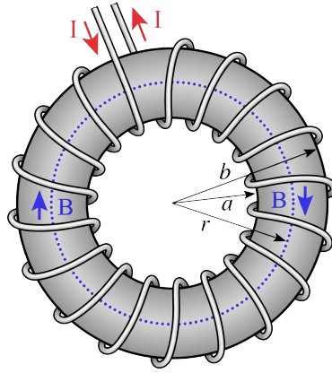
Рис. 11.10. Тороїдальна котушка
