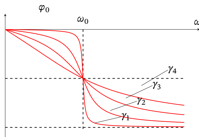
Рис. 17.6. Фазово-частотна характеристика контуру. Залежність фазового зсуву \varphi_0 від частоти \omega зовнішньої ЕРС.
