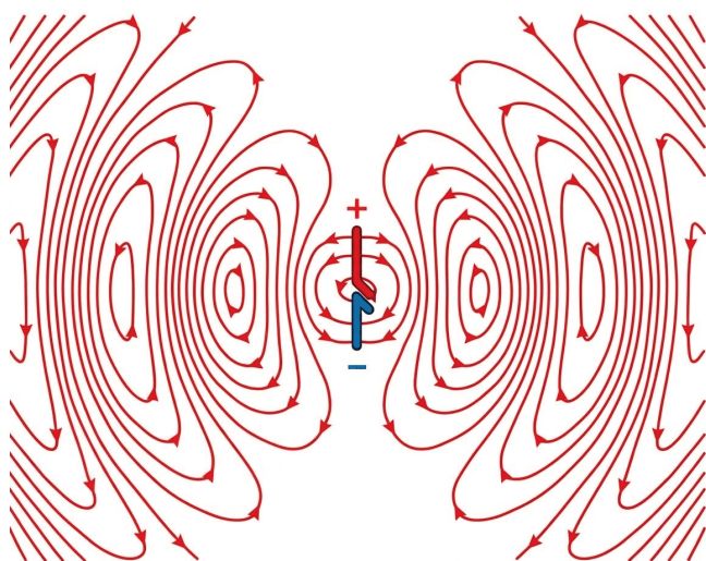
Рис. 16.7. Електричне поле осцилюючого диполя: у ближній зоні поле ніби «причеплене» до диполя, у хвильовій — випромінюється
