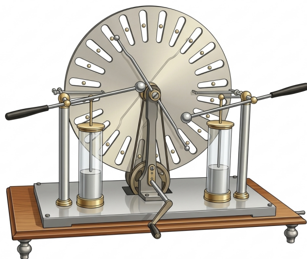
Рис. 4.4. Електрофорна машина Вімшерста: два зустрічно обертові диски з металевими секторами, схрещені нейтралізуючі стрижні, лейденські банки-конденсатори та вихідні електроди для іскрового розряду.
