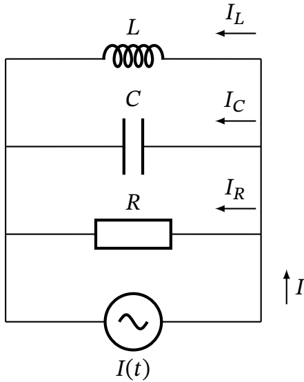
Рис. 17.10. Паралельний LCR -контур, що включає джерело заданого змінного струму I(t) = I_0 \cos \omega t .
