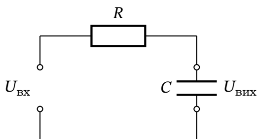
Рис. 17.15. Фільтр низьких частот: вихідна напруга знімається з конденсатора C .
