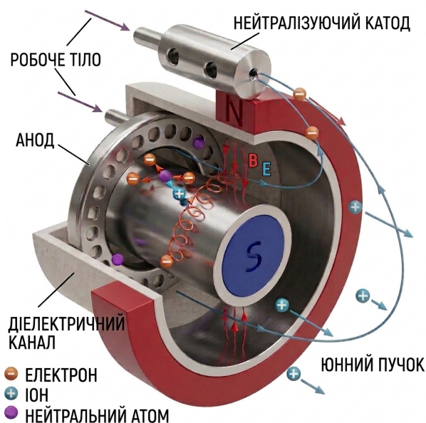
Рис. 10.6. Схема холлівського двигуна.
