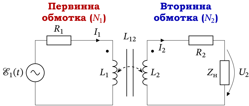
Рис. 17.13. Еквівалентна схема реального трансформатора з котушками L_1, L_2 , крапками фазування (вказують на однакову полярність виводів), активними опорами R_1, R_2 , взаємною індуктивністю L_{12} та навантаженням Z_H .
