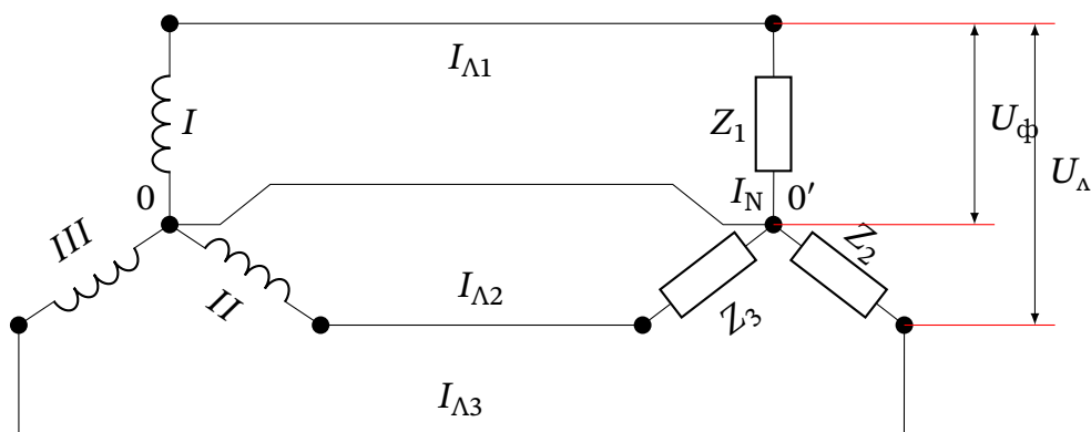
Рис. 17.21. З'єднання трифазної системи зіркою з нейтральним проводом
