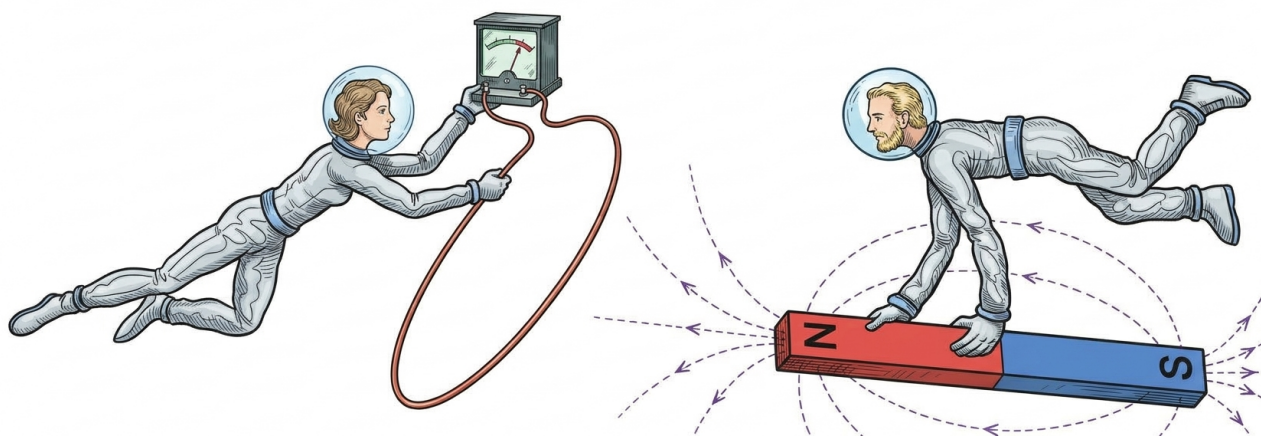
Рис. 14.1. Аліса та Боб, кожен з яких вважає нерухомим себе, по-різному пояснюють причину виникнення того самого струму в провіднику: для Аліси це електричне поле рухомого магніту, для Боба — сила Лоренца з боку магнітного поля нерухомого магніту
