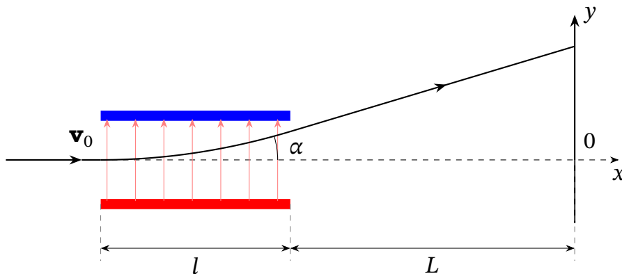
Рис. 10.7. Відхилення зарядженої частинки електричним полем конденсатора.
