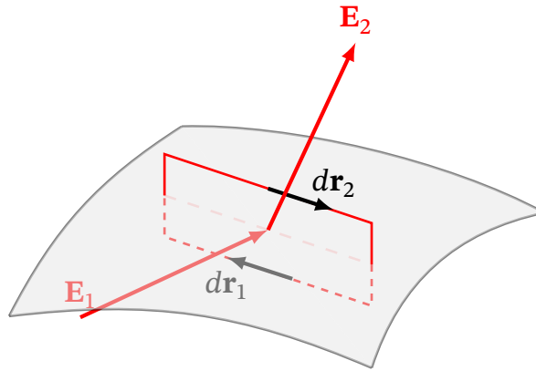
Рис. 5.9. Контур циркуляції на межі розділу двох середовищ для виведення граничної умови на тангенціальну складову \mathbf{E}
