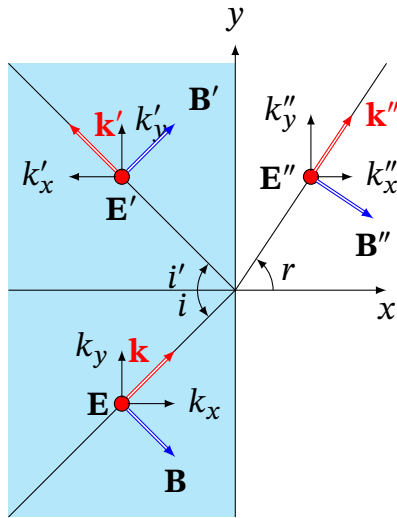
Рис. 15.8. Падаюча, відбита й заломлена s-поляризовані хвилі на межі розділу двох діелектриків
