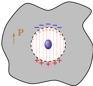
Рис. 5.11. Сферична порожнина Лоренца в поляризованому діелектрику
