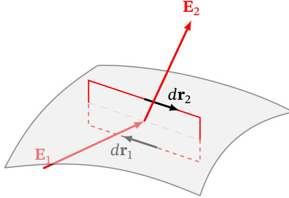
Рис. 2.22. До виведення другої граничної умови
