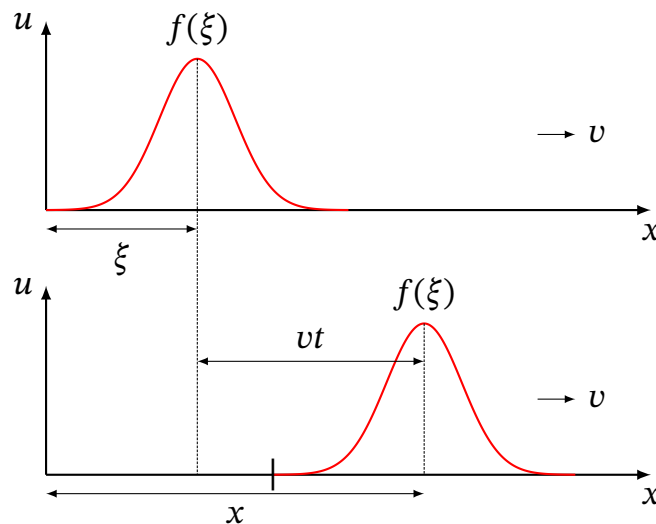
Рис. 15.2. Збурення, що поширюється без зміни форми зі швидкістю v : профіль у момент t — це профіль у момент 0, зсунутий на vt
