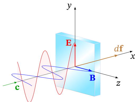
Рис. 15.5. Механізм виникнення тиску електромагнітної хвилі: сила Ампера df , що діє на струм, збуджений полем E , у полі B
