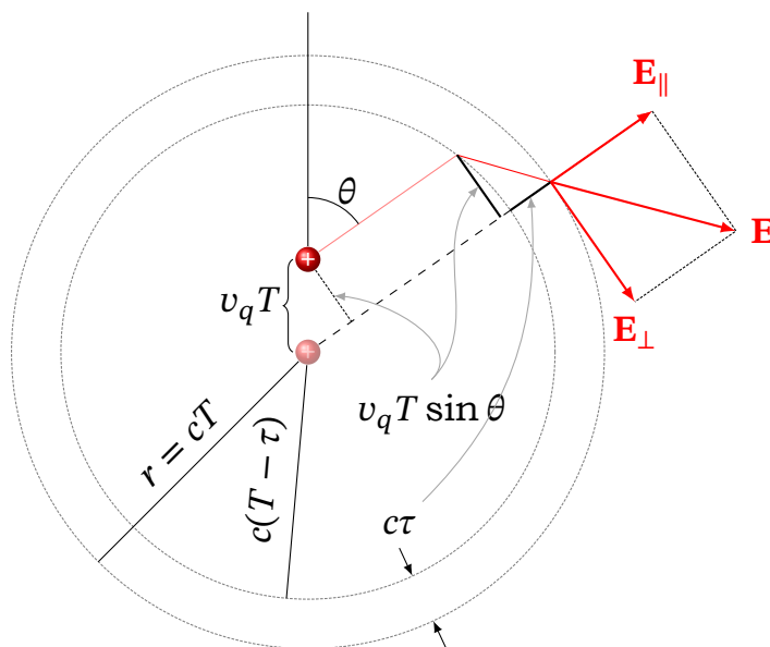
Рис. 16.4. Геометрія зламу силової лінії: розкладання поля на поздовжню E_{\parallel} і поперечну E_{\perp} складові
