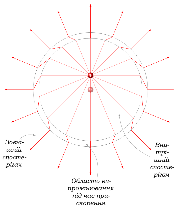
Рис. 16.3. Заломлені («злами») силові лінії поля короткочасно прискореного заряду: межа між «старим» і «новим» полем
