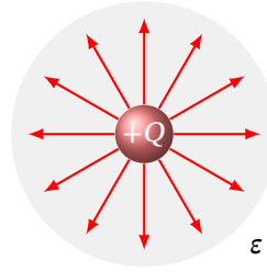
Рис. 5.7. Точковий заряд у нескінченному однорідному діелектрику
