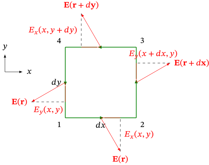
Рис. 2.19. До введення ротора через циркуляцію
