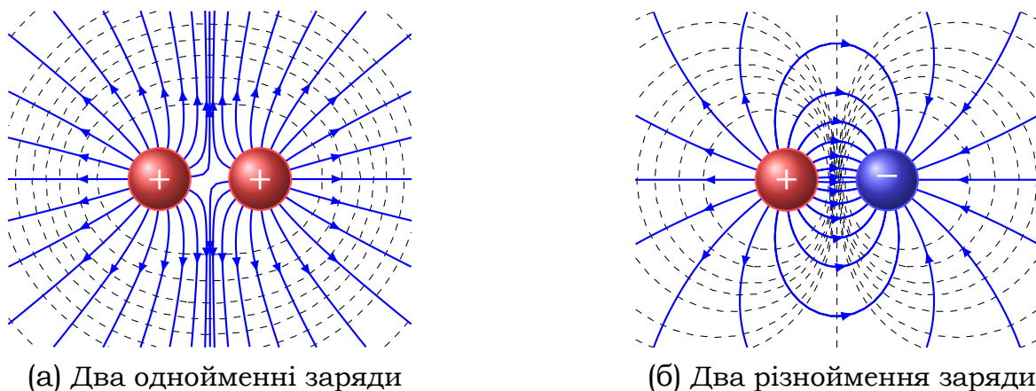
Рис. 2.6. Вигляд силових ліній системи двох зарядів
