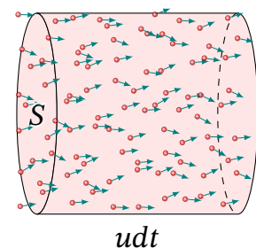
Рис. 7.2. До виведення зв'язку густини струму з дрейфовою швидкістю носіїв
