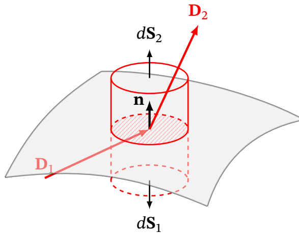
Рис. 5.8. Циліндр Гаусса на межі розділу двох середовищ для виведення граничної умови на нормальну складову \mathbf{D}
