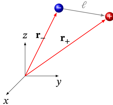
Рис. 3.1. Електричний диполь
