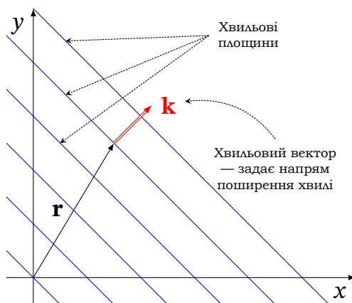
Рис. 15.3. Хвильовий вектор \mathbf{k} вказує напрям поширення плоскої хвилі й перпендикулярний до хвильових площин
