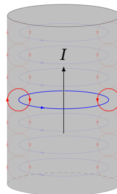
Рис. 13.7. Якісний механізм скін-ефекту: вихрові струми Фуко підсилюють струм на поверхні й послаблюють у центрі провідника
