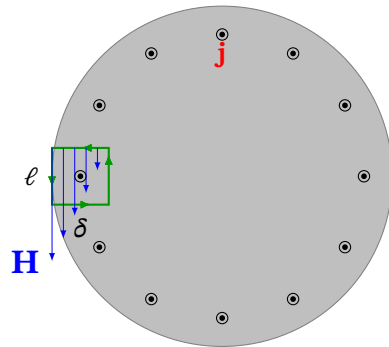
Рис. 13.9. Контур для оцінки циркуляції H поблизу поверхні провідника
