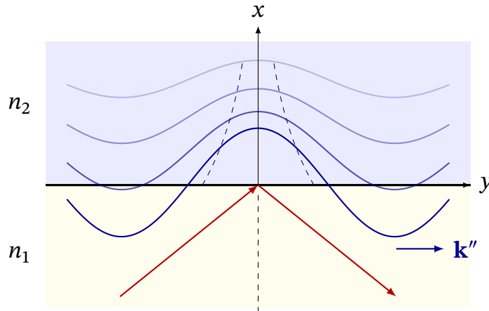
Рис. 15.11. Згасаюча хвиля в другому середовищі при i > i_b (s-поляризація:
