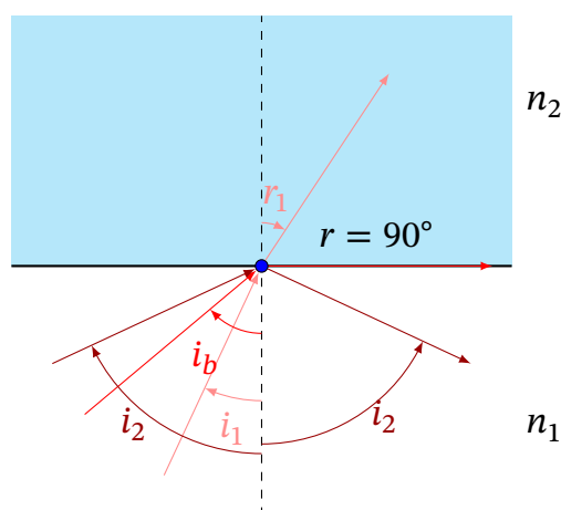
Рис. 15.10. Заломлений промінь наближається до поверхні розділу при зростанні кута падіння
