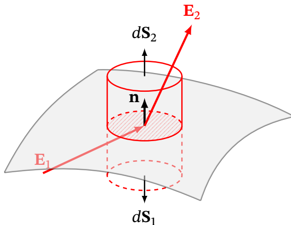
Рис. 2.21. До виведення першої граничної умови
