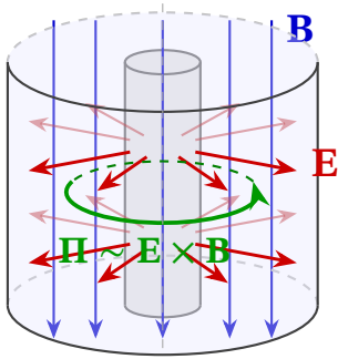
Рис. 15.7. Циліндричний конденсатор в аксіальному магнітному полі: зображено поля \mathbf{E} , \mathbf{B} і вектор Пойнтінга \mathbf{P} , що циркулює навколо осі
