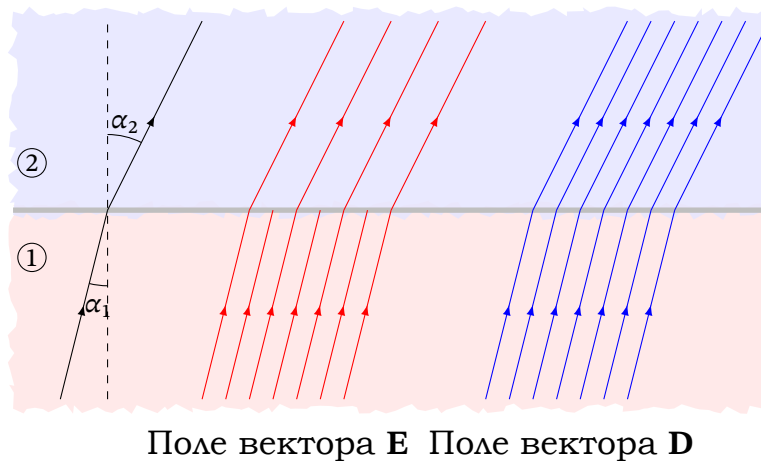
Рис. 5.10. Заломлення силових ліній \mathbf{E} і \mathbf{D} на межі розділу двох діелектриків
