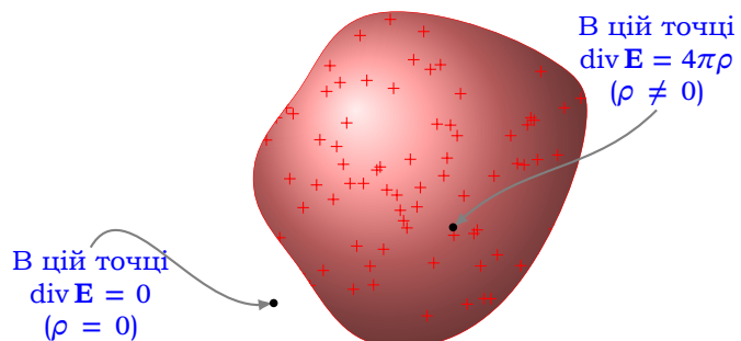
Рис. 2.13. Дивергенція поля \mathbf{E} у даній точці залежить тільки від густини електричного заряду \rho у тій самій точці і більше ні від чого.
