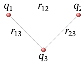
Рис. 6.4. Система трьох точкових зарядів: взаємна енергія набирається із внесків усіх пар
