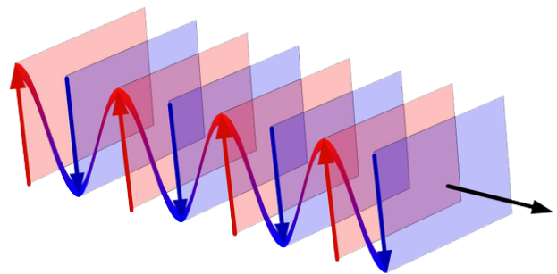
Рис. 15.3. Хвильовий вектор \mathbf{k} вказує напрям поширення плоскої хвилі й перпендикулярний до хвильових площин
