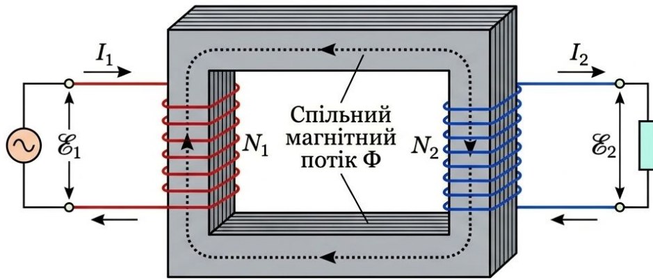
Рис. 12.6. Принципова схема трансформатора
