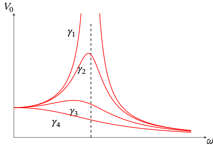
Рис. 17.5. Амплітудно-частотна характеристика контуру. Залежність амплітуди вимушених коливань V_0 від частоти \omega зовнішньої ЕРС.
