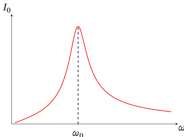
Рис. 17.9. Залежність амплітуди коливань струму від частоти коливань ЕРС — резонанс напруги на конденсаторі і ЕРС в послідовному LCR -контурі (рис. 17.1).
