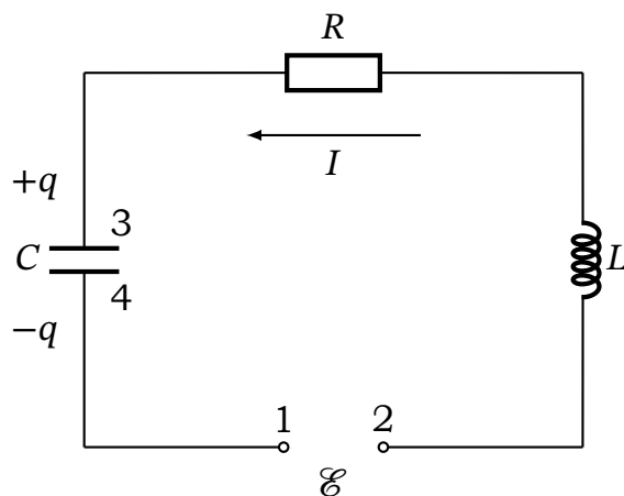
Рис. 17.1. Контур, що включає конденсатор, індуктивність, опір R і стороннє джерело ЕРС \mathcal{E} .
