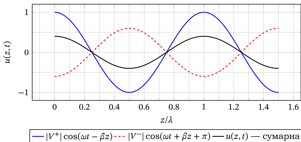
Рис. 18.2. Інтерференція падаючої та відбитої хвиль у лінії без втрат при |V^-|/|V^+| = 0.6 . Сумарна напруга утворює стоячу хвилю з вузлами та пучностями. Коефіцієнт стоячої хвилі КСХ = (1 + 0.6)/(1 - 0.6) = 4 .
