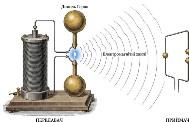
Рис. 16.1. Вібратор Герца.
