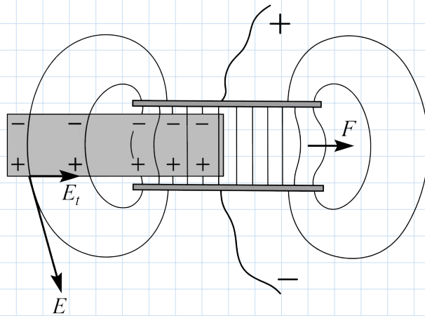
Рис. 6.7. Модель конденсатора з частково всунутою пластиною діелектрика: паралельне з'єднання вакуумного та заповненого діелектриком конденсаторів
