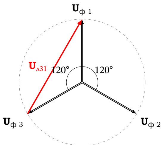
Рис. 17.22. Векторна діаграма співвідношення фазних та лінійних напруг
