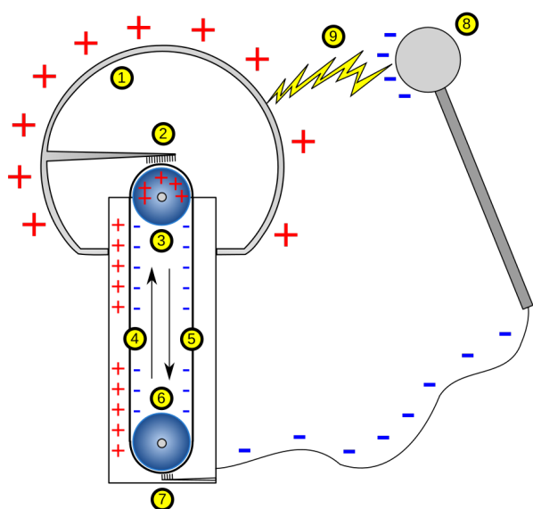
Рис. 4.8. Генератор Ван-де-Граафа
