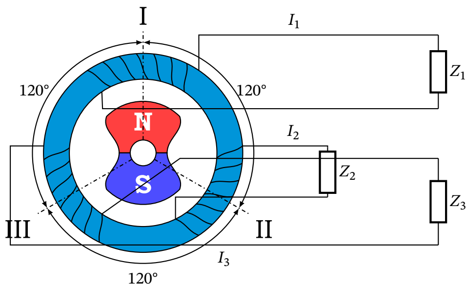
Рис. 17.19. Схематичне зображення трифазного синхронного генератора
