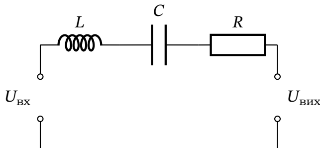
Рис. 17.17. Смуговий фільтр на основі послідовного LCR -контур: вихідна напруга знімається з резистора R .
