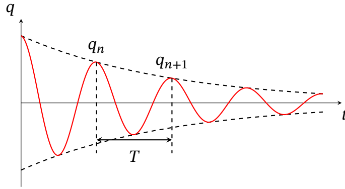
Рис. 17.4. Затухаючі коливання. До означення логарифмічного декременту.
