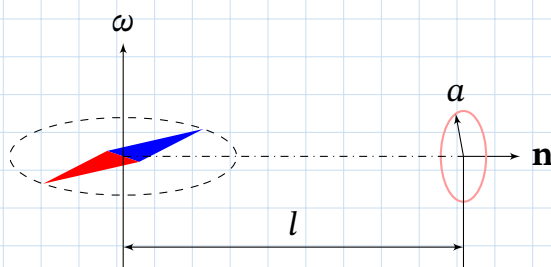
Рис. 12.5. Магнітний диполь, що обертається, і нерухоме кільце на відстані \ell
