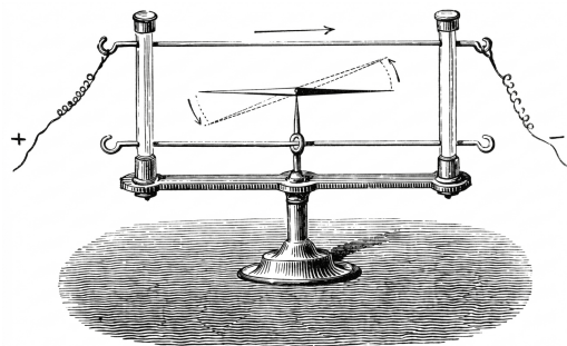
Рис. 8.1. Установка Ерстеда
