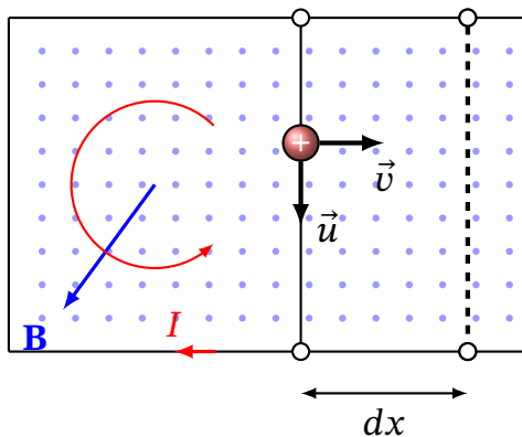
Рис. 11.3. Виникнення ЕРС індукції в рухомій перемичці: на позитивний заряд + у провіднику, що рухається зі швидкістю \mathbf{v} , діє сила Лоренца \mathbf{F}_L , напрямлена вздовж провідника (швидкість \mathbf{u} ). Ця сила викликає індукційний струм I у контурі
