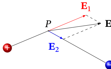
Рис. 2.3. Ілюстрація принципу суперпозиції для випадку двох різноіменних зарядів
