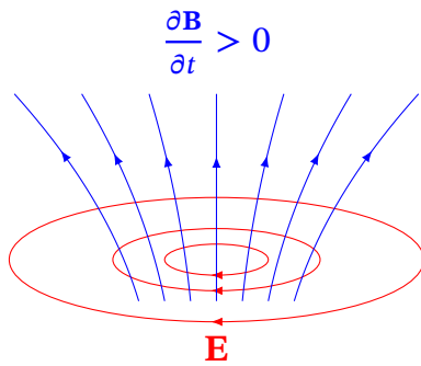
Рис. 11.8. Вихрове електричне поле, породжене зростаючим у часі магнітним полем
