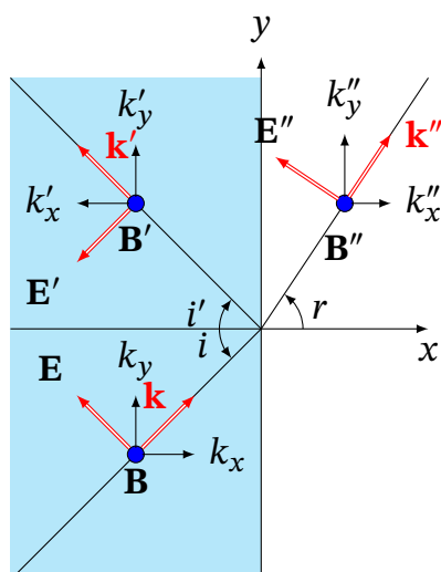
Рис. 15.9. Падаюча, відбита й заломлена p -поляризовані хвилі на межі розділу двох діелектриків
