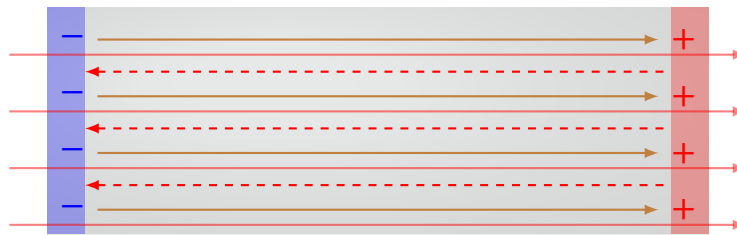
Рис. 5.5. Поляризований діелектрик у зовнішньому електричному полі: на поверхнях виникають зв'язані заряди -Q та +Q . Стрілки означають: \rightarrow — зовнішнє поле \mathbf{E}_{\text{ex}} ; \leftarrow — поле зв'язаних зарядів \mathbf{E}' ; \rightarrow — вектор поляризації \mathbf{P} (також співпадає з результуючим полем \mathbf{E} ).
