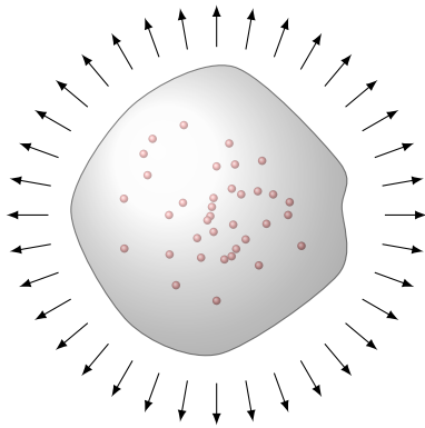
Рис. 13.5. Заряджені частинки в області, обмеженій замкненою поверхнею: енергія електромагнітного поля може втікати й витікати крізь цю поверхню
