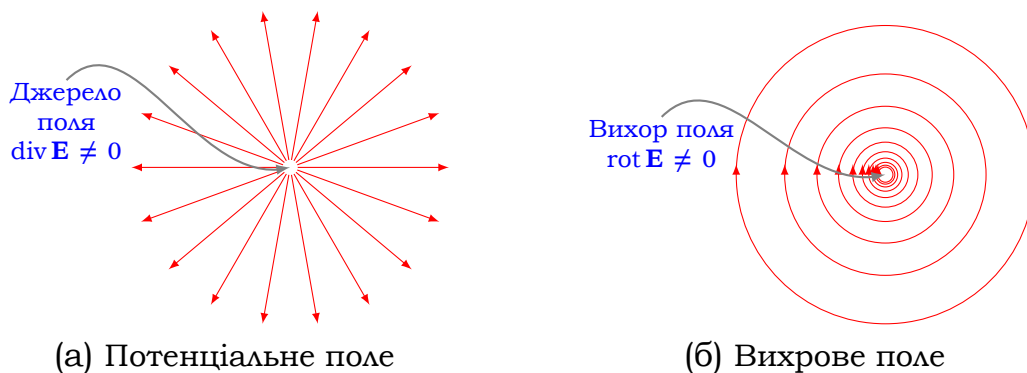
Рис. 2.20. Приклад силових ліній потенціального та вихрового полів
