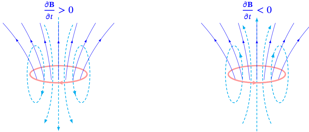
Рис. 11.6. Правило Ленца: напря́м індукційного струму залежить від знака \partial \mathbf{B} / \partial t
