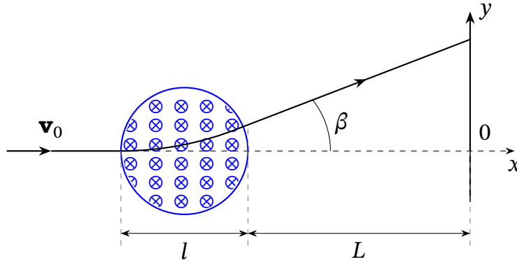
Рис. 10.8. Відхилення зарядженої частинки магнітним полем.
