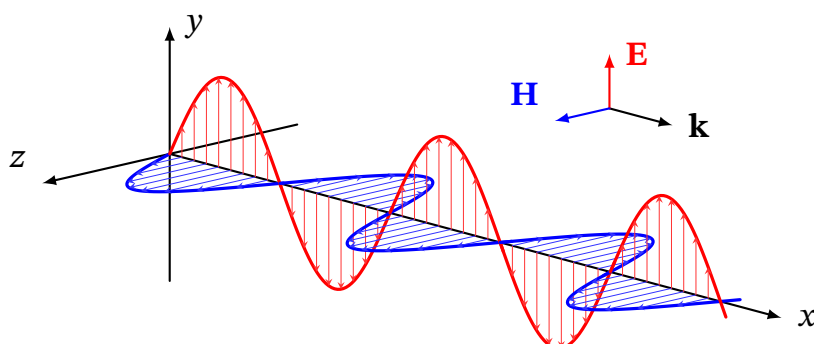
Рис. 15.4. Плоска монохроматична електромагнітна хвиля: взаємно перпендикулярні коливання \mathbf{E} і \mathbf{H} , що поширюються вздовж \mathbf{k}
