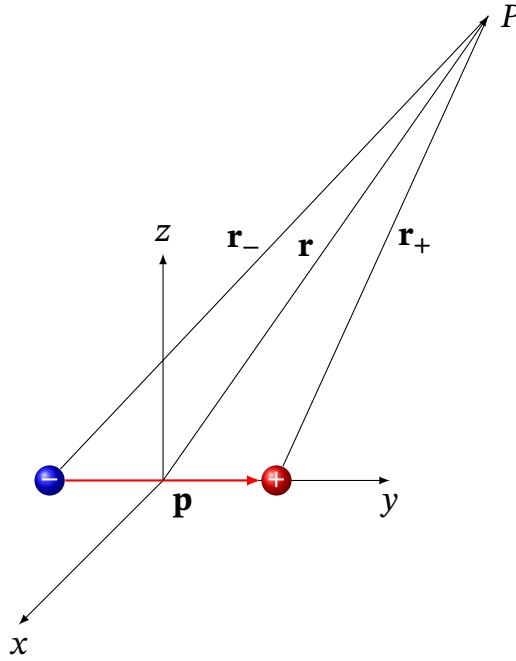
Рис. 3.2. До виведення напруженості та потенціалу поля диполя
