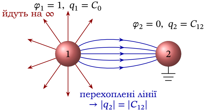
Рис. 6.1. Частина силових ліній провідника 1 замикається на заземленому провіднику 2, решта йде на нескінченність
