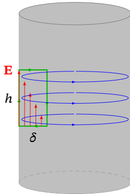
Рис. 13.8. Контур для оцінки циркуляції E поблизу поверхні провідника
