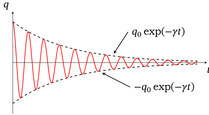
Рис. 17.3. Графік затухаючих коливань. Штриховою лінією показано часову залежність амплітуди A(t) = q_0 e^{-\gamma t} .
