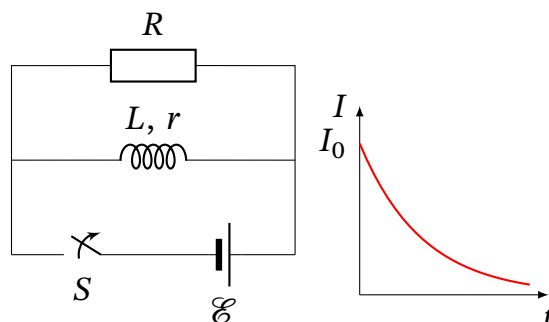
Рис. 11.12. Екстраструм розмикання в колі з індуктивністю
