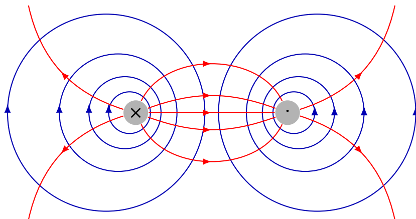
Рис. 18.4. Лінії електричного (червоні) та магнітного (сині) полів для біжучої хвилі в перерізі двопровідної лінії
