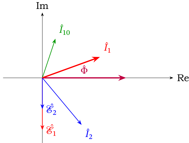
Рис. 17.14. Векторна діаграма трансформатора в режимі навантаження. Потік \hat{\Phi} напрямлений уздовж дійсної осі; ЕРС відстають від нього на \pi/2 ; струм \hat{I}_1 є сумою струму холостого ходу та скомпенсованого вторинного струму.
