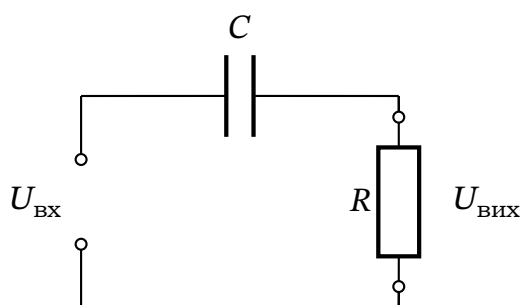
Рис. 17.16. Фільтр високих частот: вихідна напруга знімається з резистора R .
