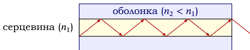
Рис. 19.3. Поширення світла в оптичному волокні завдяки повному внутрішньому відбиттю на межі серцевина–оболонка: промінь «замкнений» усередині серцевини й рухається вздовж волокна майже без втрат.
