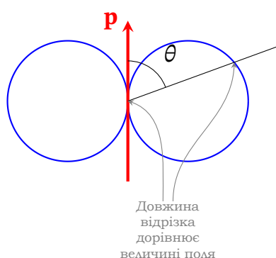
Рис. 16.8. Полярна діаграма спрямованості дипольного випромінювача: характерна форма «бублика»
