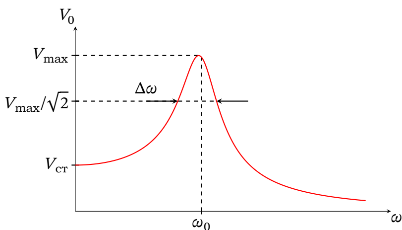
Рис. 17.7. Характеристики резонансної кривої: V_{\text{max}} — максимум амплітуди, V_{\text{ст}} — статична амплітуда, \Delta\omega — ширина резонансу.
