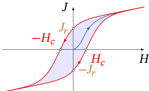
Рис. 9.11. Петля гістерезису феромагнетика: J_r — залишкова намагніченість, H_c — коерцитивна сила
