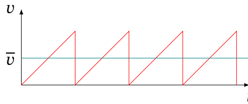
Рис. 8.1. Пилкоподібна залежність швидкості електрона від часу в моделі Друде
