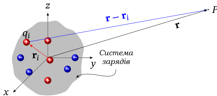
Рис. 3.3. До визначення потенціалу на далеких відстанях
