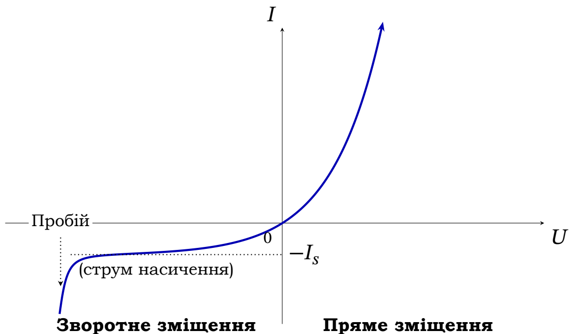
Рис. 8.17. Вольт-амперна характеристика p - n -переходу
