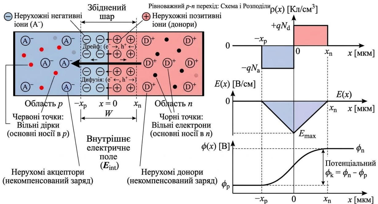
Рис. 8.16. Рівноважний p - n -перехід
