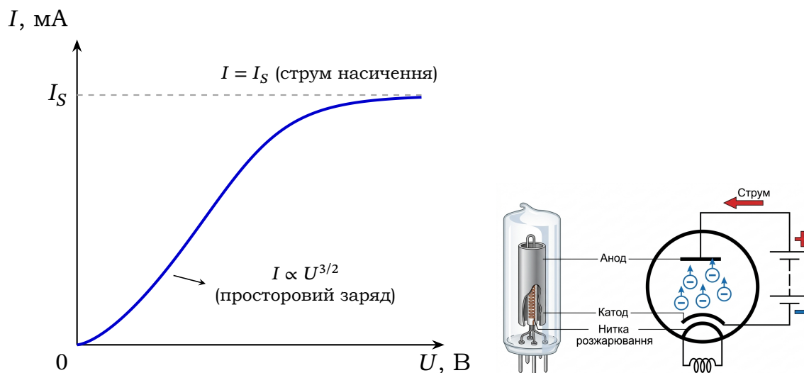
Рис. 8.12. Вольт-амперна характеристика вакуумного діода
