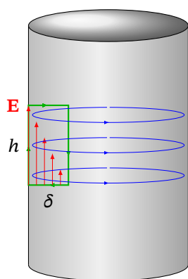
Рис. 14.9. Контур для оцінки циркуляції \mathbf{E} поблизу поверхні циліндричного провідника (вигляд збоку)
