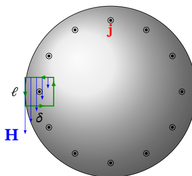
Рис. 14.10. Контур для оцінки циркуляції \mathbf{H} поблизу циліндричної поверхні провідника (вигляд зверху)
