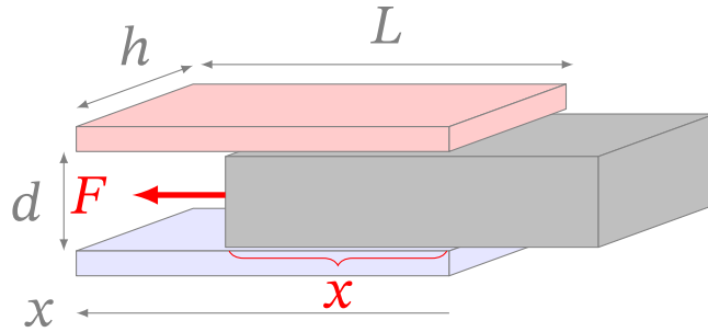
Рис. 6.6. Модель конденсатора з частково всунутою пластинною діелектрика: паралельне з'єднання вакуумного та заповненого діелектриком конденсаторів
