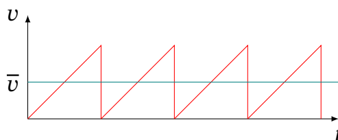
Рис. 7.6. Пилкоподібна залежність швидкості електрона від часу в моделі Друде
