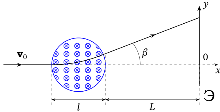
Рис. 12.6. Відхилення зарядженої частинки магнітним полем. М — магніт, Е — екран. Напрямок магнітного поля перпендикулярно площині листа і направлено «за лист».
