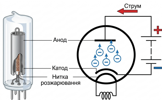
Рис. 8.12. Вигляд вакуумного діода: нагрітий катод емітує електрони, які прискорюються до анода під дією електричного поля. При зміні полярності анода струм не проходить.
