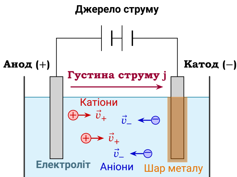
Рис. 8.6. Електроліз: рух йонів у розчині й осадження речовини на катоді
