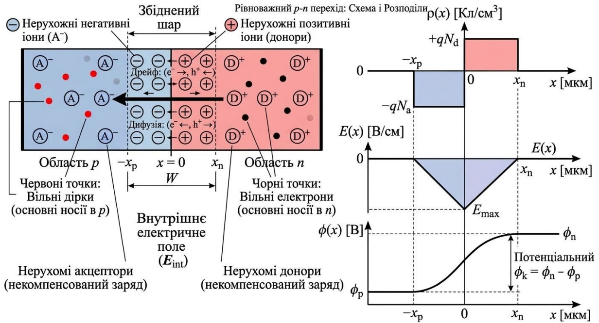
Рис. 8.18. Рівноважний p - n -перехід
