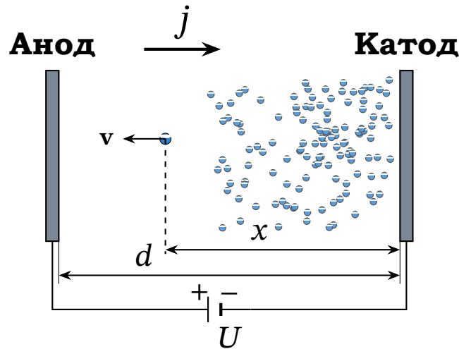
Рис. 8.13. Розподіл просторового заряду та електронів у плоскому вакуумному діоді.
