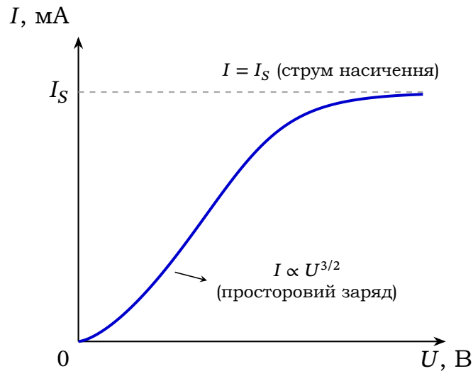
Рис. 8.14. Вольт-амперна характеристика вакуумного діода
