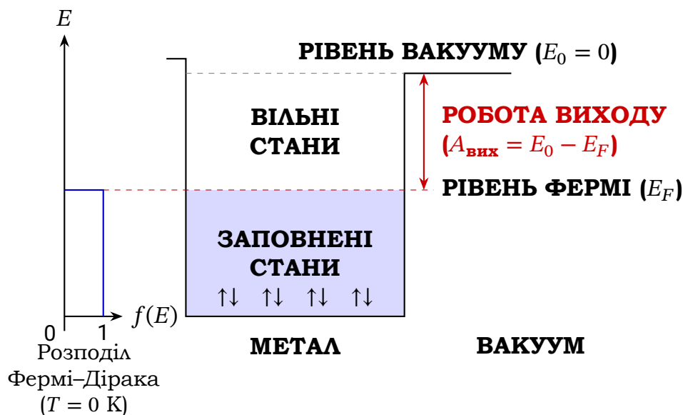
Рис. 8.11. Потенціальна яма електрона в металі: рівень Фермі, рівень вакууму, робота виходу A_{\text{вих}} ; заповнені стани електронів
