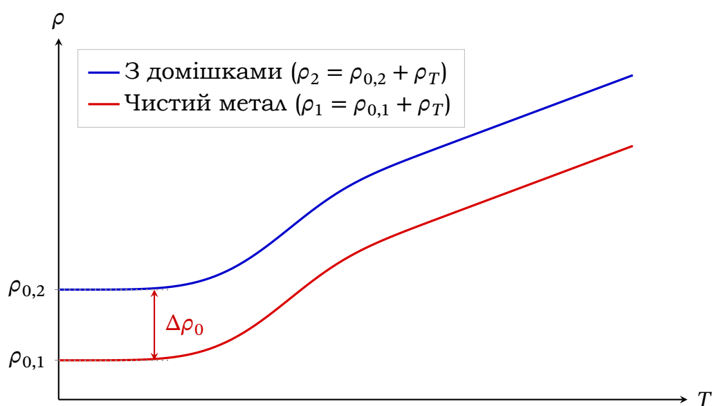
Рис. 8.3. Правило Маттіссена: домішки додають до опору сталу \rho_0 , не змінюючи температурної частини
