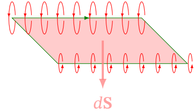
Рис. 10.4. Довільний замкнений контур L у намагніченій речовині
