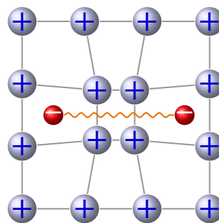
Рис. 8.5. Утворення куперівської пари через обмін фононами
