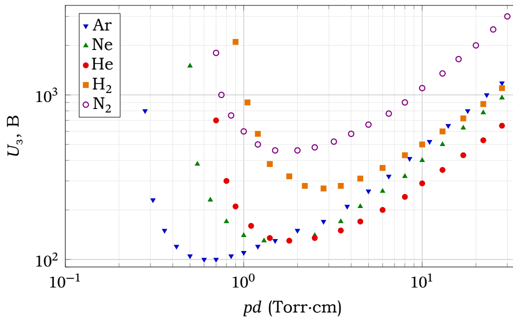
Рис. 8.9. Закон Пашена
