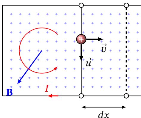
Рис. 12.3. Виникнення ЕРС індукції в рухомій перемичці: на позитивний заряд + у провіднику, що рухається зі швидкістю \mathbf{v} , діє сила Лоренца \mathbf{F}_L , спрямована вздовж провідника (швидкість \mathbf{u} ). Ця сила викликає індукційний струм I у контурі
