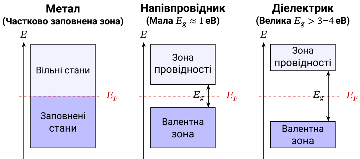
Рис. 8.15. Зонна структура металу, напівпровідника й діелектрика
