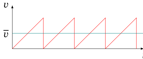
Рис. 8.1. Пілкоподібна залежність швидкості електрона від часу в моделі Друде
