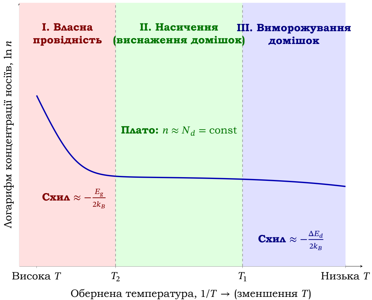
Рис. 8.17. Три температурні області провідності домішкового напівпровідника
