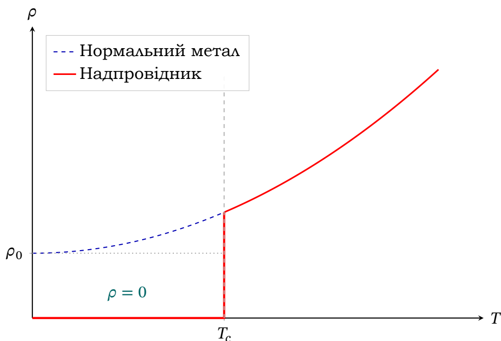
Рис. 8.4. Характерна залежність питомого опору від температури металу, який переходить в надпровідний: при високих T — майже лінійне зростання, T < T_c опір стрибкоподібно падає до нуля
