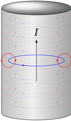
Рис. 14.8. Якісний механізм скін-ефекту: вихрові струми Фуко підсилюють струм на поверхні й послаблюють у центрі провідника
