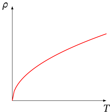
Рис. 8.2. Передбачення найпростішої теорії Друде: \rho \propto \sqrt{T}
