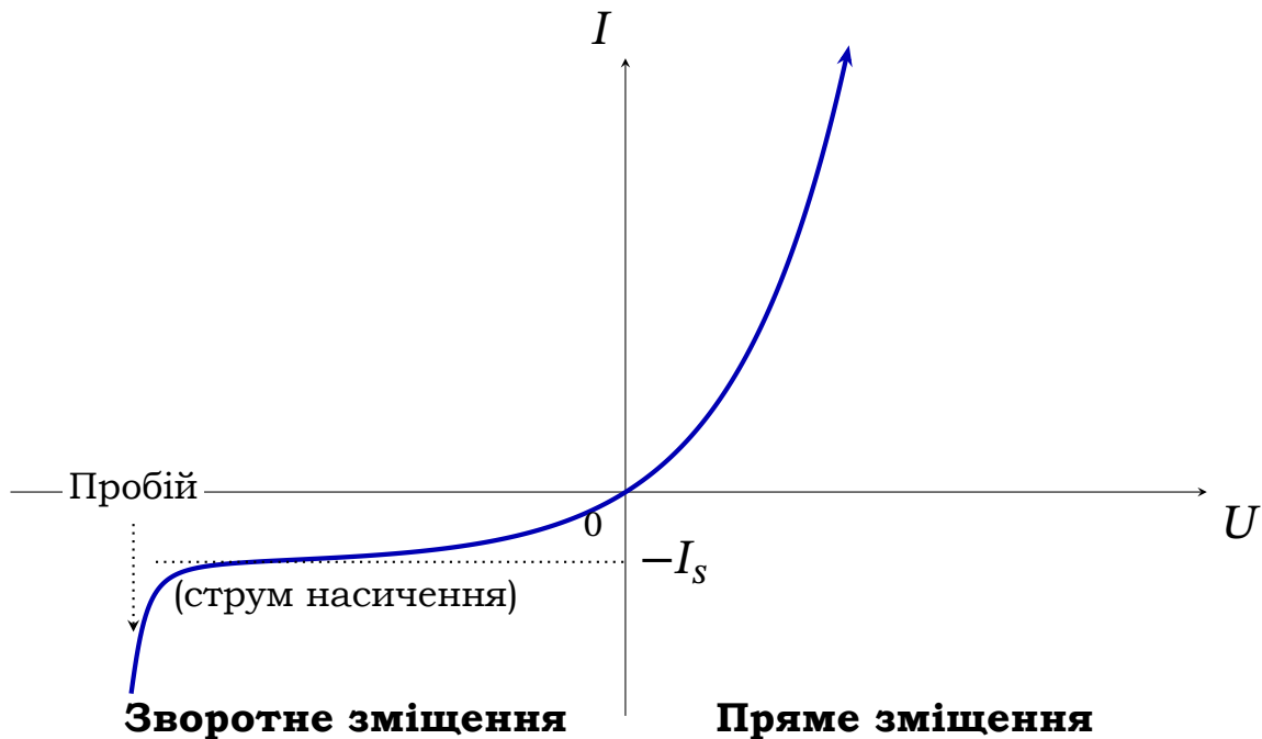
Рис. 8.19. Вольтамперна характеристика p - n -переходу
