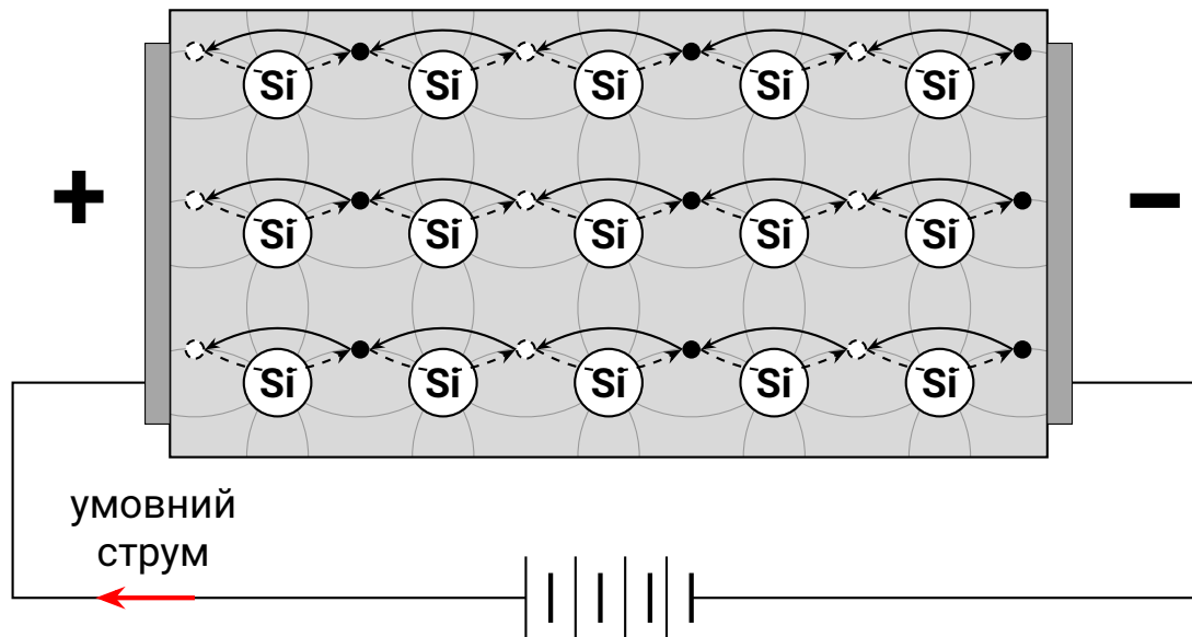
Рис. 8.16. Рух дірки як естафета електронів на сусідні вакансії. Електрони позначені чорними кружками, дірки — білими. Дірки рухаються праворуч, електрони — ліворуч.
