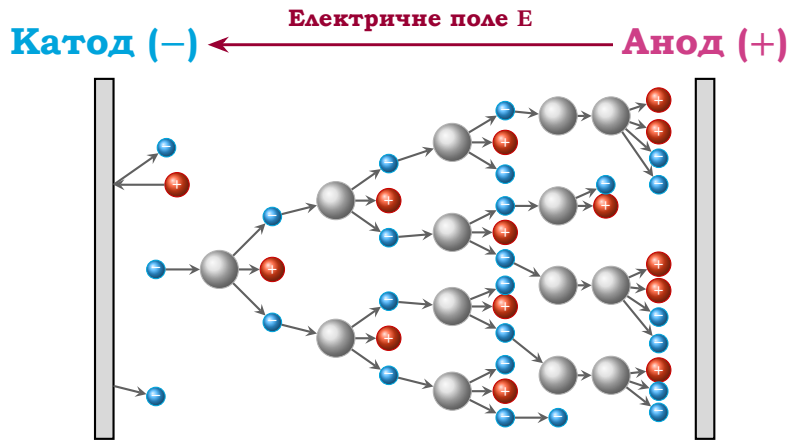
Рис. 8.8. Електронна лавина та вторинна емісія з катода
