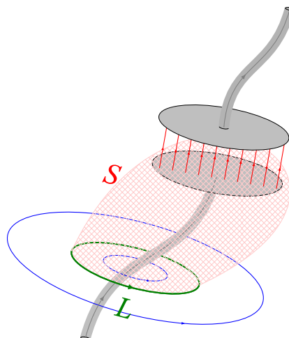
Рис. 14.2. Контур L , натягнута на нього поверхня S та провідник зі струмом, що її пронизує
