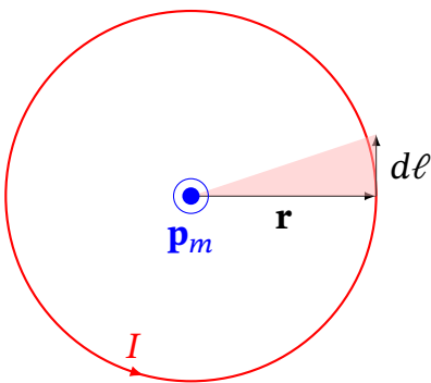
Рис. 9.13. До обчислення магнітного моменту колового витка зі струмом
