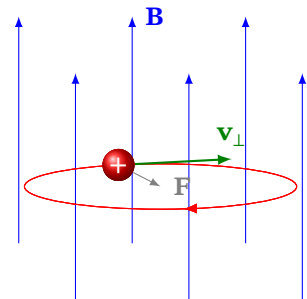
Рис. 9.5. Кругова траєкторія зарядженої частинки в однорідному магнітному полі: сила завжди перпендикулярна до швидкості
