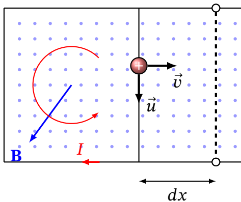
Рис. 10.3. Виникнення ЕРС індукції в рухомій перемичці: на позитивний заряд + у провіднику, що рухається зі швидкістю \mathbf{v} , діє сила Лоренца \mathbf{F}_{\Lambda} , напрямлена вздовж провідника (швидкість \mathbf{u} ). Ця сила викликає індукційний струм I у контурі
