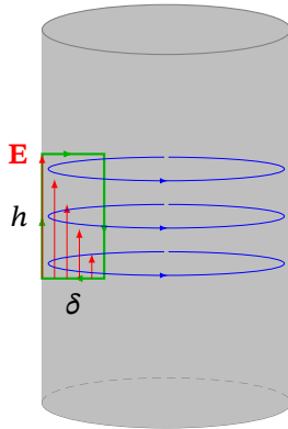
Рис. 11.12. Контур для оцінки циркуляції \mathbf{E} поблизу поверхні провідника
