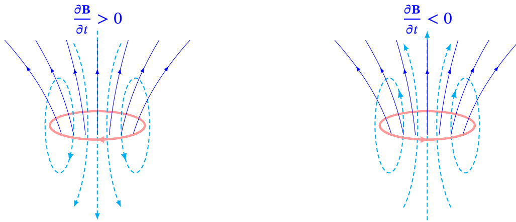
Рис. 10.6. Правило Ленца: напрям індукційного струму залежить від знака \partial B/\partial t
