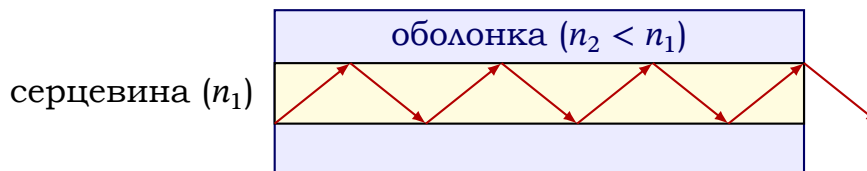
Рис. 17.3. Поширення світла в оптичному волокні завдяки повному внутрішньому відбиттю на межі серцевина–оболонка: промінь «замкнений» усередині серцевини й рухається вздовж волокна майже без втрат.
