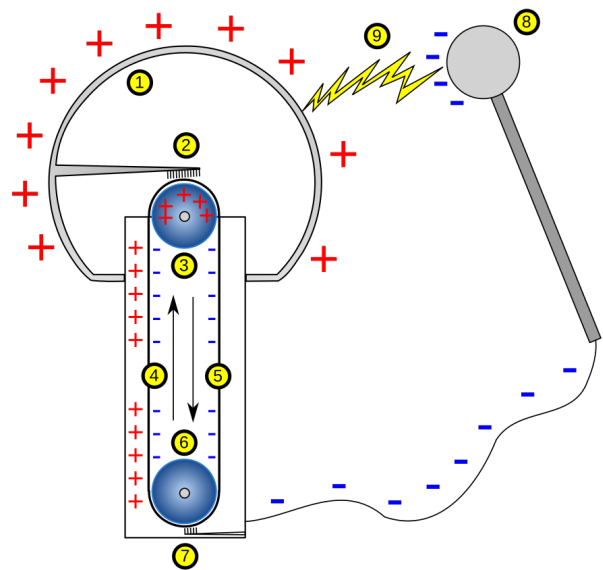
Рис. 4.8. Генератор Ван-де-Граафа
