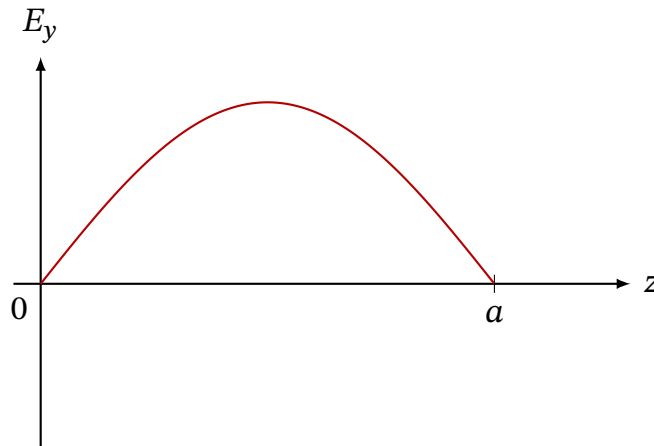
Рис. 17.2. Графік рівняння (17.3) при n = 1 .
