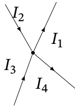
Рис. 7.11. Вузол розгалуженого кола:
