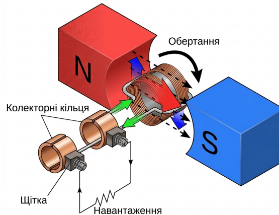
Рис. 10.4. Схема найпростішого генератора змінного струму
