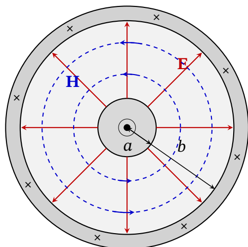
Рис. 16.4. Структура електромагнітного поля в поперечному перерізі довгої лінії (коаксіального кабелю): вектор \mathbf{E} напрямлений від внутрішньої жили до зовнішнього екрана, а лінії вектора \mathbf{H} охоплюють провідник зі струмом.
