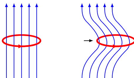
Рис. 10.8. Збереження магнітного потоку в надпровідному контурі: при переміщенні контуру в магнітному полі силові лінії, що пронизують його, залишаються «вмороженими», тобто їхня кількість не змінюється.
