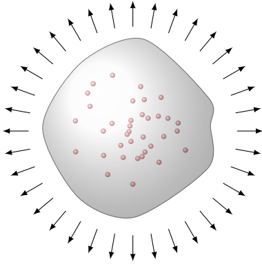
Рис. 11.7. Заряджені частинки в області, обмеженій замкнутою поверхнею: енергія електромагнітного поля може втікати й витікати крізь цю поверхню
