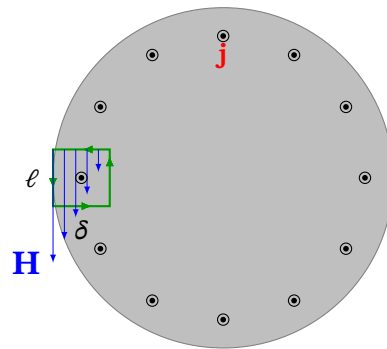
Рис. 11.13. Контур для оцінки циркуляції \mathbf{H} поблизу поверхні провідника
