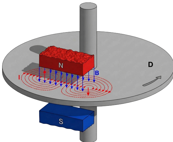
Рис. 10.7. Індукування вихрових струмів Фуко в провідному диску, що обертається в полі магніту
