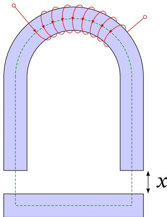
Рис. 10.20. Електромагніт з якорем, відокремленим повітряним зазором x
