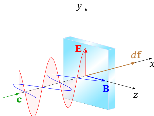
Рис. 13.5. Механізм виникнення тиску електромагнітної хвилі: сила Ампера d\mathbf{f} , що діє на струм, збуджений полем \mathbf{E} , у полі \mathbf{B}
