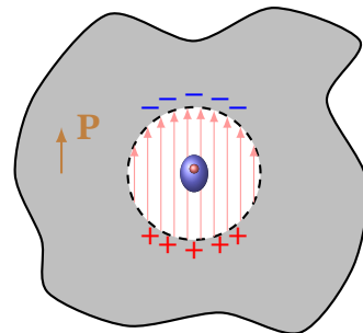
Рис. 5.12. Сферична порожнина Лоренца в поляризованому діелектрику
