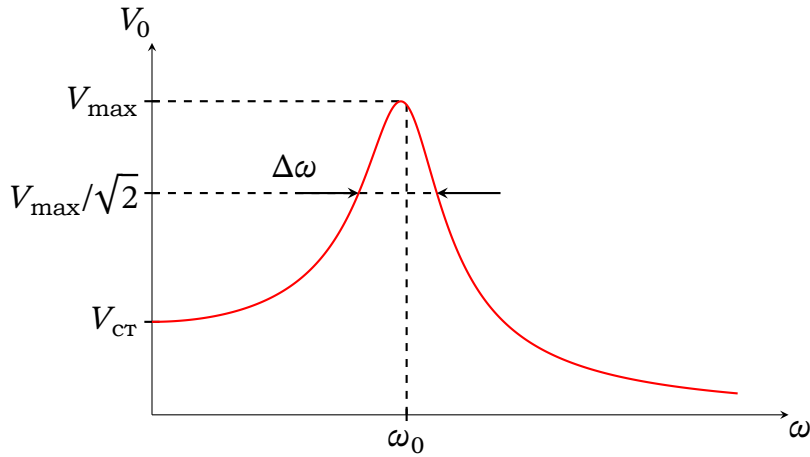
Рис. 15.6. Характеристики резонансної кривої: V_{\max} — максимум амплітуди, V_{\text{ст}} — статична амплітуда, \Delta\omega — ширина резонансу.
