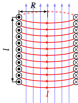
Рис. 10.18. Поздовжній переріз довгого соленоїда: однорідне поле всередині, струм у витках обмотки
