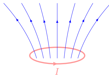
Рис. 12.10. Контур зі струмом I і створюване ним власне магнітне поле
