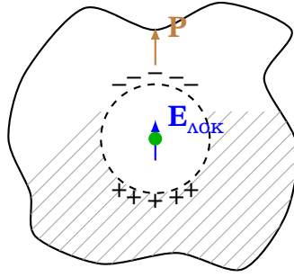
Рис. 6.1. Сферична порожнина Лоренца в поляризованому діелектрику
