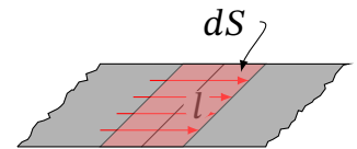
Поверхневий струм \mathbf{i} dS
