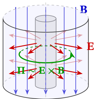
Рис. 15.8. Циліндричний конденсатор в аксіальному магнітному полі: зображено поля \mathbf{E} , \mathbf{B} і вектор Пойнтінга \mathbf{\Pi} , що циркулює навколо осі
