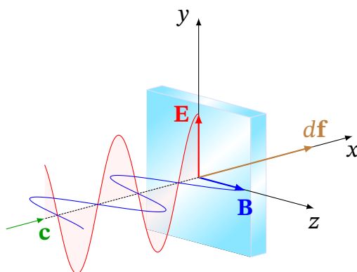
Рис. 15.5. Механізм виникнення тиску електромагнітної хвилі: сила Ампера df , що діє на струм, збуджений полем \mathbf{E} , у полі \mathbf{B}
