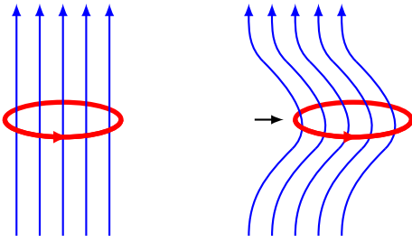
Рис. 11.12. Замороження магнітного потоку в надпровідному кільці при зміні його положення в зовнішньому полі: кільце підтримує колишній потік незгасаючим струмом
