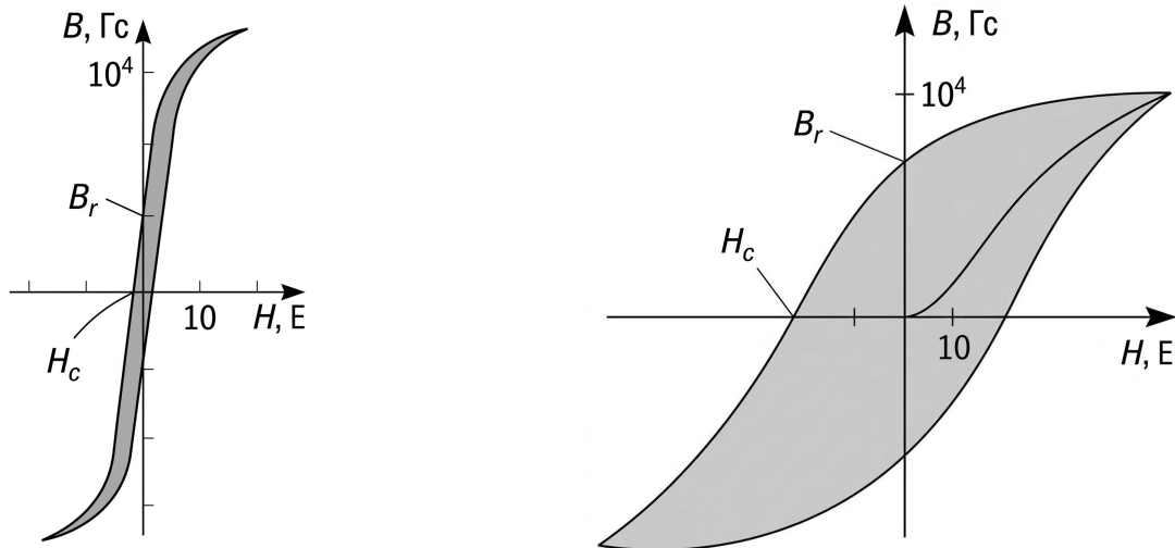
(а) Вузька петля гістерезису магнітом'якого матеріалу
