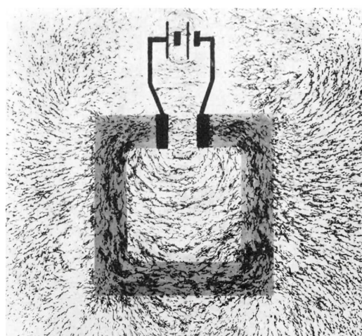
Рис. 7.9. Дослід із дрібнодисперсним порошком (фотографія з Jefimenko O. D. Demonstration of the Electric Fields of Current-Carrying Conductors // American Journal of Physics. 1962. Vol. 30, no. 1. P. 19–21).
