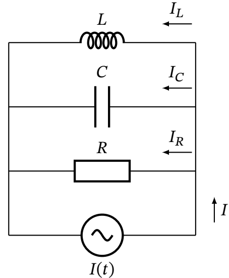
Рис. 17.10. Паралельний LCR -контур, що включає джерело заданого змінного струму I(t) = I_m \cos \omega t .
