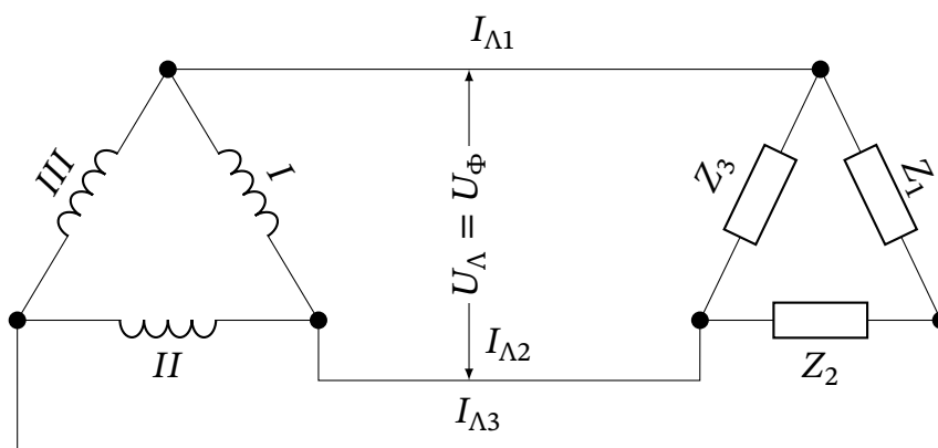
Рис. 17.23. Схема з'єднання генератора та приймача трикутником
