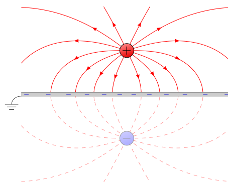
(б) Заряд над площиною та його зображення.
