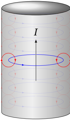
Рис. 13.8. Якісний механізм скін-ефекту: вихрові струми Фуко підсилюють струм на поверхні й послаблюють у центрі провідника
