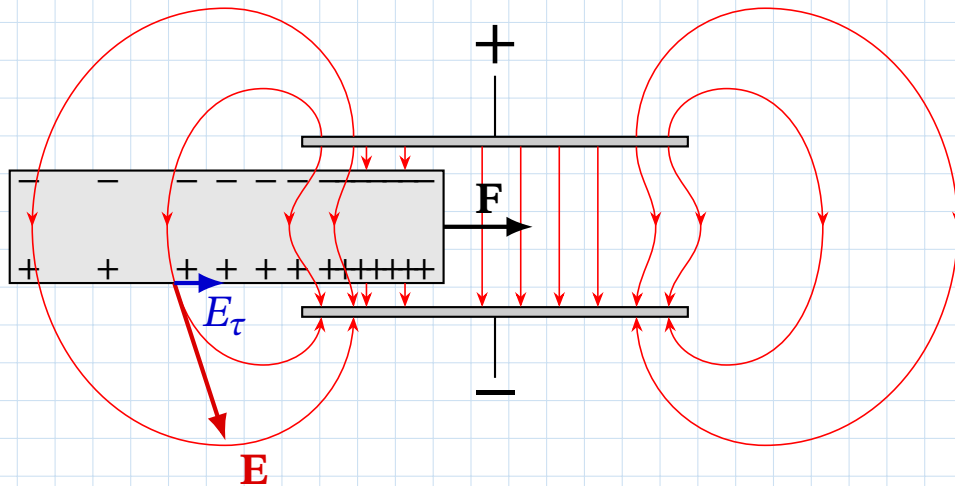
Рис. 6.7. Модель конденсатора з частково всунутою пластиною діелектрика: паралельне з'єднання вакуумного та заповненого діелектриком конденсаторів
