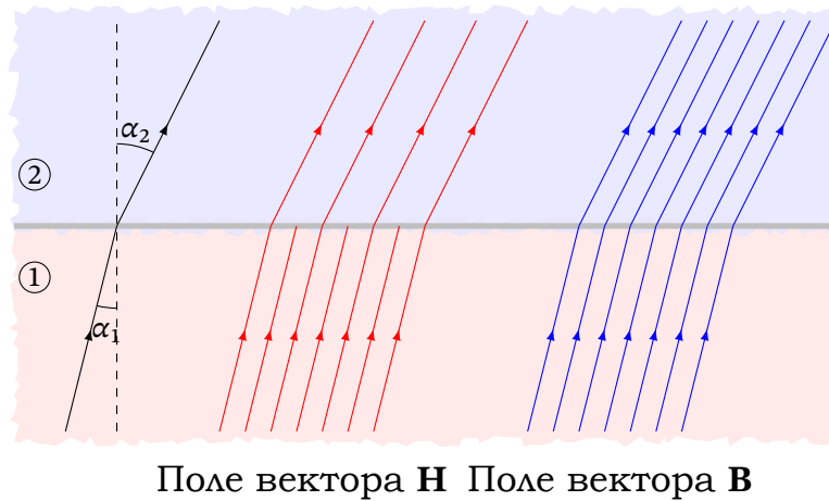
Рис. 9.7. Заломлення силових ліній H і B на межі розділу двох магнетиків
