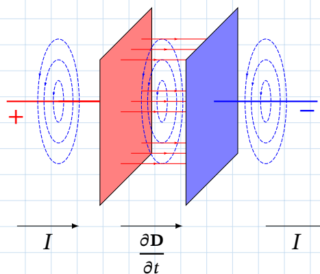
Рис. 13.3. Магнітне поле, створене струмом зміщення всередині конденсатора під час його зарядки
