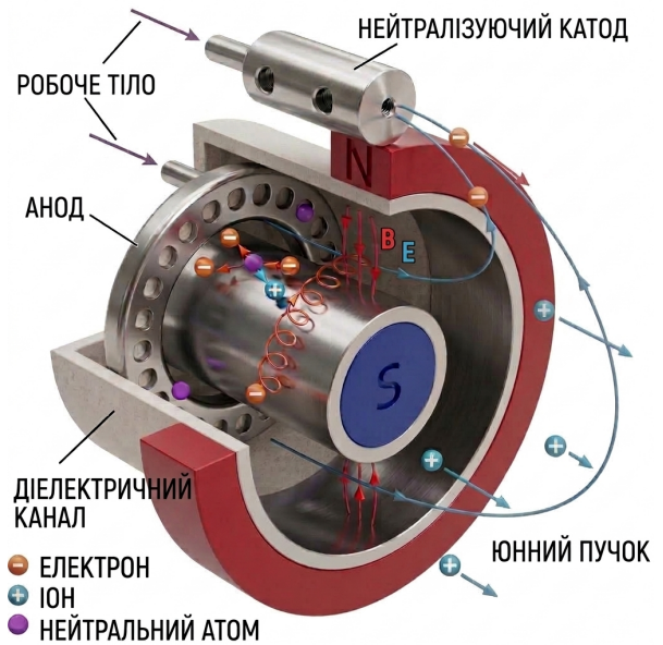
Рис. 10.6. Схема холлівського двигуна.
