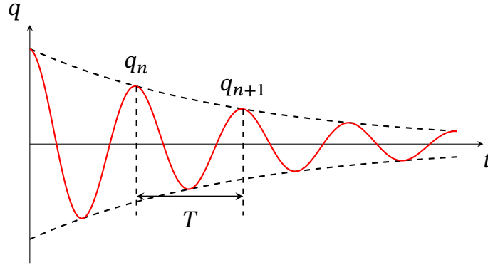
Рис. 17.4. Затухаючі колювання. До означення логарифмічного декременту.
