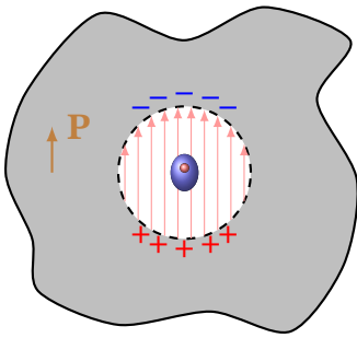
Рис. 5.11. Сферична порожнина Лоренца в поляризованому діелектрику
