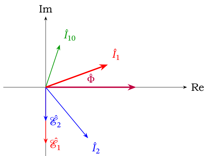
Рис. 17.14. Векторна діаграма трансформатора в режимі навантаження. Потік \Phi напрямлений уздовж дійсної осі; ЕРС відстають від нього на \pi/2 ; струм \hat{I}_1 є сумою струму холостого ходу та скомпенсованого вторинного струму.
