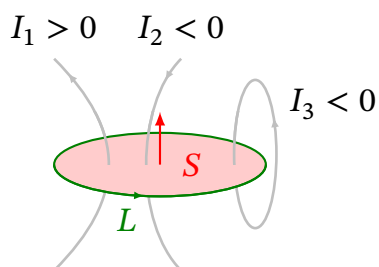
Рис. 8.10. Струм враховують зі знаком «плюс», якщо його напрям узгоджений із напрямом обходу контуру L за правилом правого гвинта, і зі знаком «мінус» — у протилежному випадку
