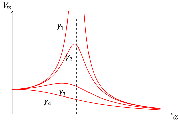
Рис. 17.5. Амплітудно-частотна характеристика контуру. Залежність амплітуди вимушених коливань V_m від частоти \omega зовнішньої ЕРС.
