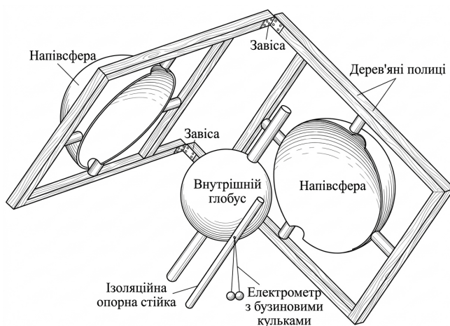
Рис. 1.5. Установа Г. Кавендіша для перевірки закону обернених квадратів.
