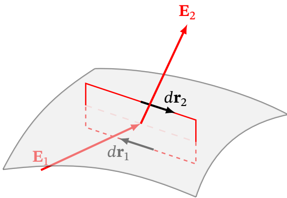
Рис. 5.9. Контур циркуляції на межі розділу двох середовищ для виведення граничної умови на тангенціальну складову E
