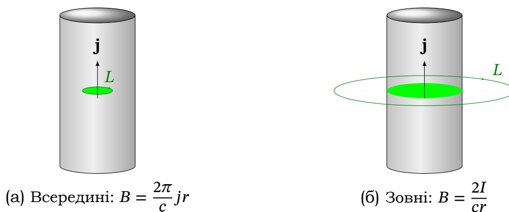
Рис. 8.12. Поле нескінченного циліндричного провідника зі струмом: усередині й поза провідником
