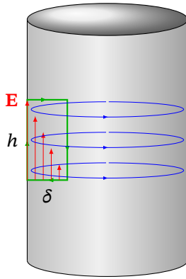
Рис. 13.9. Контур для оцінки циркуляції \mathbf{E} поблизу поверхні циліндричного провідника (вигляд збоку)
