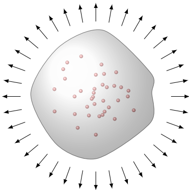
Рис. 13.6. Заряджені частинки в області, обмеженій замкненою поверхнею: енергія електромагнітного поля може втікати й витікати крізь цю поверхню
