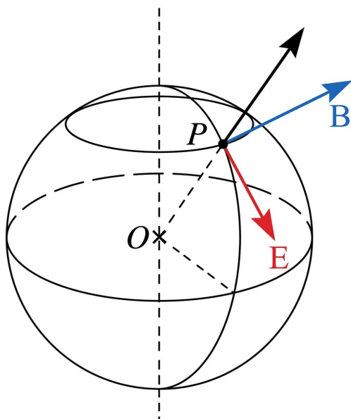
Рис. 16.6. Поля E_\theta і B_\varphi у хвильовій зоні диполя
