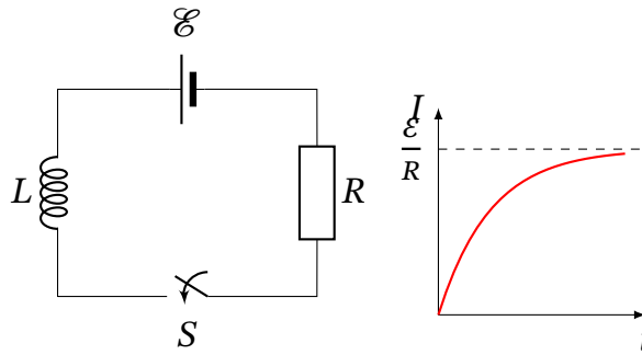
Рис. 11.10. Встановлення струму в колі з індуктивністю після замикання ключа
