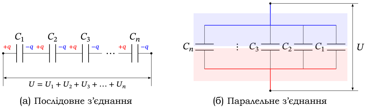
Рис. 6.3. З'єднання конденсаторів: (а) послідовне — заряд на всіх обкладках однаковий, напруги додаються; (б) паралельне — напруга на всіх конденсаторах однакова, заряди додаються
