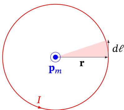
Рис. 8.13. До обчислення магнітного моменту колового витка зі струмом
