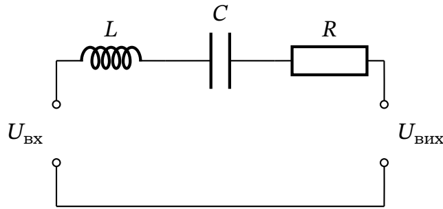
Рис. 17.17. Смуговий фільтр на основі послідовного LCR -контуру: вихідна напруга знімається з резистора R .
