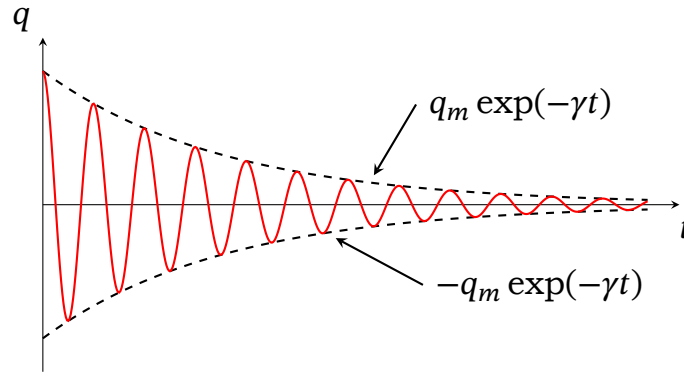
Рис. 17.3. Графік затухаючих коливань. Штриховою лінією показано часову залежність амплітуди A(t) = q_m e^{-\gamma t} .
