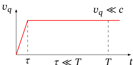
Рис. 16.2. Швидкість заряду: короткий імпульс прискорення тривалістю \tau , після якого заряд рухається рівномірно
