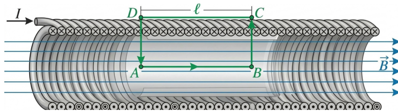
Рис. 8.11. До розрахунку магнітного поля нескінченно довгого соленоїда.
