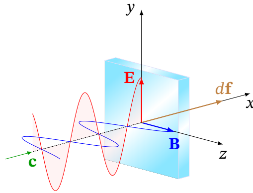
Рис. 15.5. Механізм виникнення тиску електромагнітної хвилі: сила Ампера df , що діє на струм, збуджений полем E , у полі B
