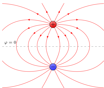
(а) Конфігурація поля двох різнойменних зарядів.
