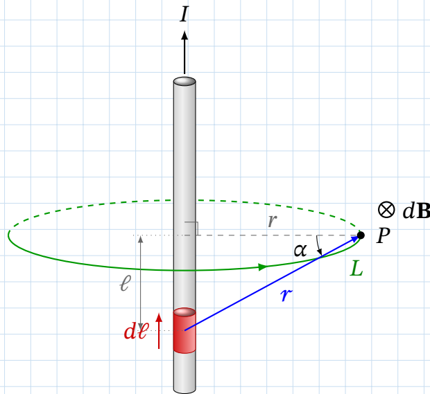
Рис. 8.7. До обчислення магнітного поля нескінченного провідника зі струмом.
