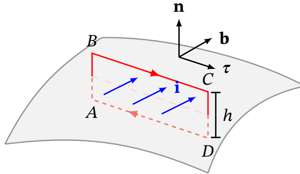
Рис. 9.6. Контур циркуляції на межі розділу двох магнетиків
