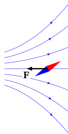
Рис. 8.16. Магнітний диполь у неоднорідному полі втягується в область сильнішого поля
