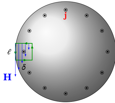
Рис. 13.10. Контур для оцінки циркуляції \mathbf{H} поблизу циліндричного поверхні провідника (вигляд зверху)
