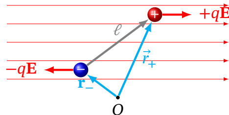
Рис. 3.4. до виведення моменту сил, що діє на диполь в однорідному електричному полі
