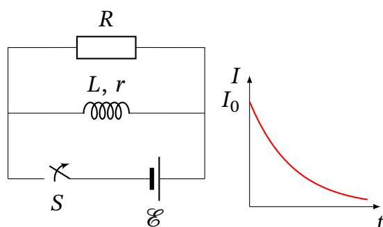
Рис. 11.11. Екстраструм розмикання в колі з індуктивністю
