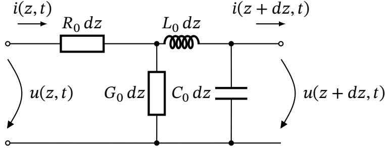
Рис. 18.1. Схема заміщення елементарного відрізка довгої лінії як чотириполосника. Паралельні елементи G_0 dz і C_0 dz рознесені для наочності.
