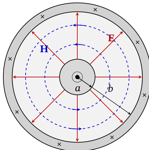
Рис. 16.4. Структура електромагнітного поля в поперечному перерізі довгої лінії (коаксiального кабелю): вектор \mathbf{E} напрямлений від внутрішньої жили до зовнішнього екрана, а лінії вектора \mathbf{H} охоплюють провідник зі струмом.
