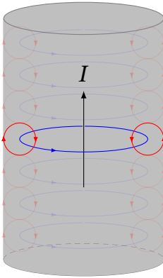
Рис. 11.11. Якісний механізм скін-ефекту: вихрові струми Фуко підсилюють струм на поверхні й послаблюють у центрі провідника
