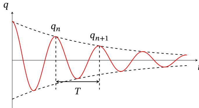
Рис. 15.3. Затухаючі колювання. До означення логарифмічного декременту.
