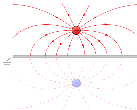
(б) Заряд над площиною та його зображення.
