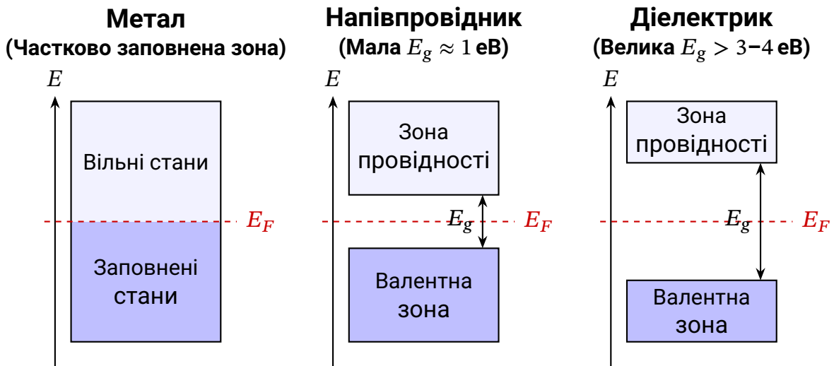
Рис. 8.13. Зонна структура металу, напівпровідника й діелектрика
