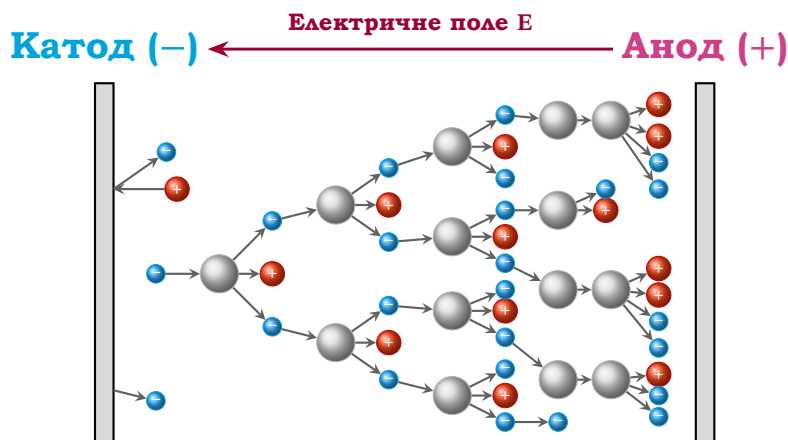
Рис. 8.7. Електронна лавина та вторинна емісія з катода
