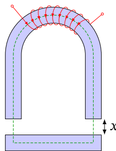
Рис. 10.20. Електромагніт з якорем, відокремленим повітряним зазором x
