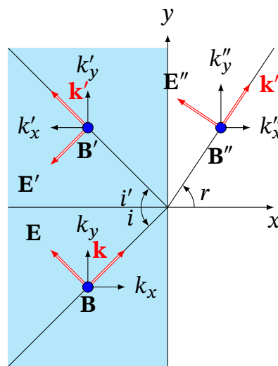
Рис. 12.9. Падаюча, відбита й заломлена p -поляризовані хвилі на межі розділу двох діелектриків
