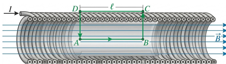
Рис. 8.11. До розрахунку магнітного поля нескінченно довгого соленоїда.
