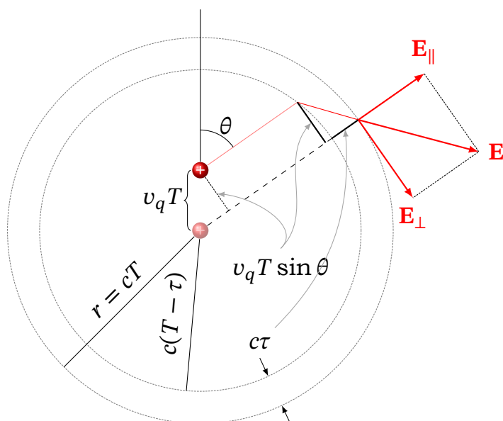
Рис. 17.4. Геометрія зламу силової лінії: розкладання поля на поздовжню E_{\parallel} і поперечну E_{\perp} складові
