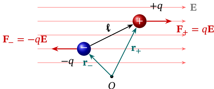
Рис. 3.4. до виведення моменту сил, що діє на диполь в однорідному електричному полі
