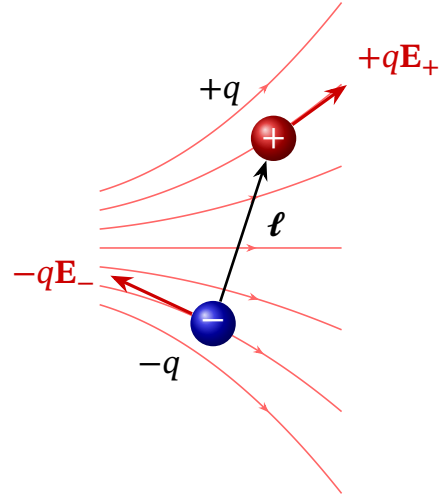
Рис. 3.5. Диполь у неоднорідному полі
