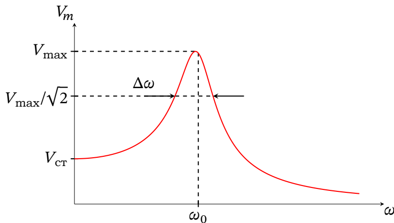
Рис. 18.7. Характеристики резонансної кривої: V_{\text{max}} — максимум амплітуди, V_{\text{ст}} — статична амплітуда, \Delta\omega — ширина резонансу.
