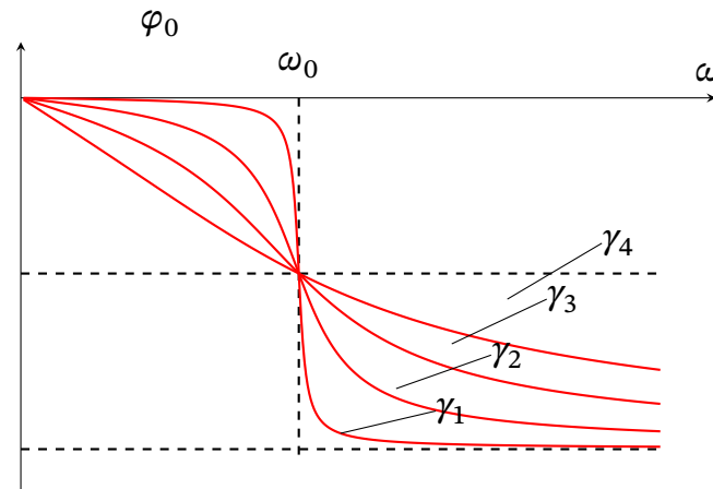
Рис. 18.6. Фазово-частотна характеристика контуру. Залежність фазового зсуву \varphi_0 від частоти \omega зовнішньої ЕРС.
