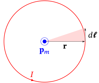
Рис. 9.13. До обчислення магнітного моменту колового витка зі струмом
