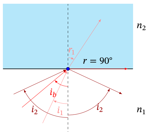
Рис. 16.11. Заломлений промінь наближається до поверхні розділу при зростанні кута падіння
