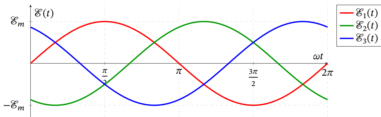
Рис. 18.20. Часові діаграми симетричної трифазної системи ЕРС
