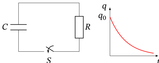
Рис. 7.16. Розрядка конденсатора через резистор: коло та графік q(t)
