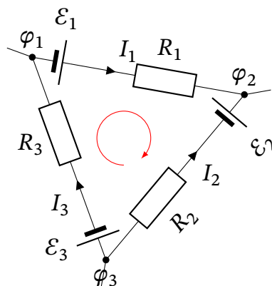
Рис. 7.13. Контур розгалуженого кола з трьома ЕРС і трьома резисторами
