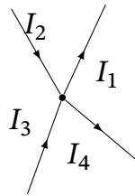
Рис. 7.12. Вузол розгалуженого кола: I_1 + I_4 = I_2 + I_3
