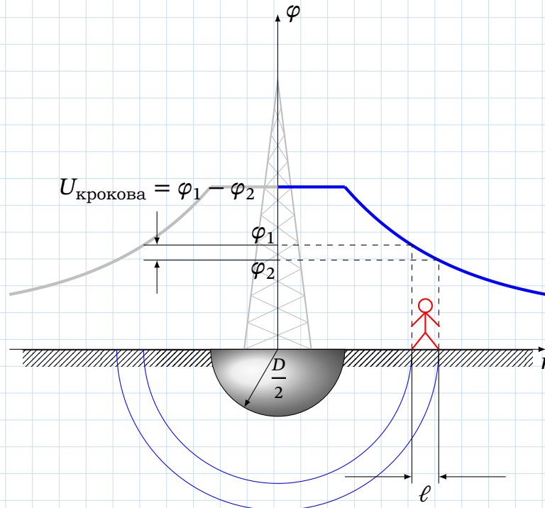
Рис. 7.15. Розтікання струму від напівсферичного заземлювача та крокова напруга
