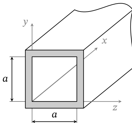
Рис. 19.1. Прямокутний хвильовід
