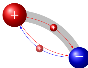
Рис. 7.10. У замкненому колі частина носіїв мусить рухатися проти сил електростатичного поля — це можливо лише завдяки стороннім силам
