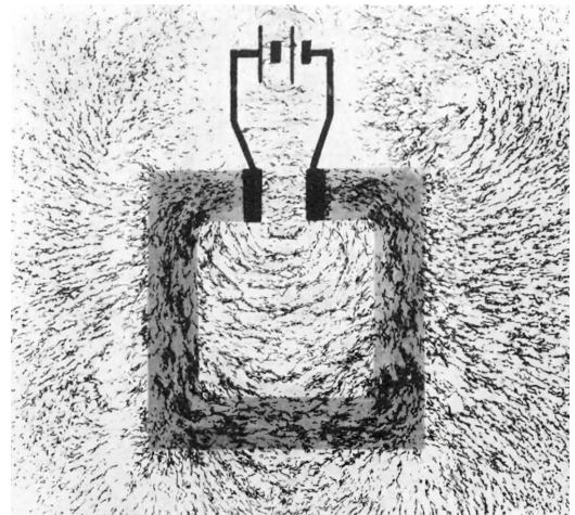
Рис. 7.9. Дослід із дрібнодисперсним порошком (фотографія з Jefimenko O. D. Demonstration of the Electric Fields of Current-Carrying Conductors // American Journal of Physics. 1962. Vol. 30, no. 1. P. 19–21).
