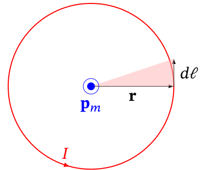
Рис. 8.13. До обчислення магнітного моменту колового витка зі струмом
