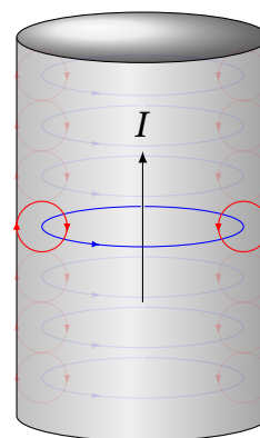
Рис. 13.8. Якісний механізм скін-ефекту: вихрові струми Фуко підсилюють струм на поверхні й послаблюють у центрі провідника
