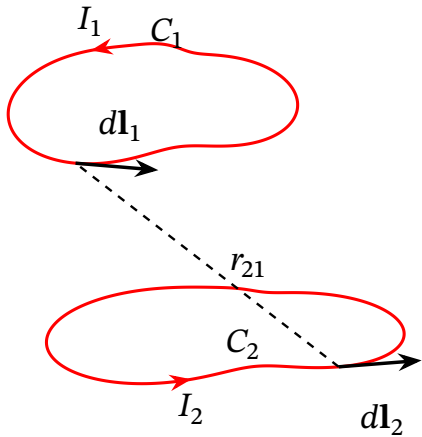
Рис. 12.3. До доведення теореми взаємності. Зображено контури C_1 і C_2 , елементи d\mathbf{l}_1 , d\mathbf{l}_2 та радіус-вектор \mathbf{r}_{21} між ними, які використовуються при обчисленні потоку \Phi_{12} .
