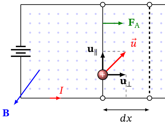
Рис. 11.2. Рамка з рухомою перемичкою в магнітному полі: показано силу Ампера F_A , що діє на перемичку зі струмом I , зміщення dx та розклад повної швидкості \vec{u} носія заряду на складові \vec{u}_\perp (рух разом із перемичкою) і \vec{u}_\parallel (рух уздовж провідника)
