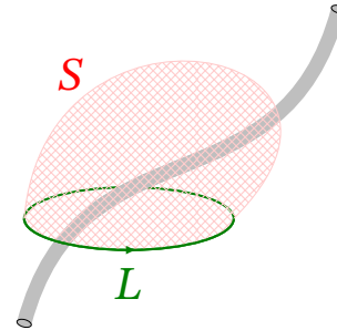
Рис. 8.9. Контур L і натягнута на нього поверхня S , крізь яку протікає струм
