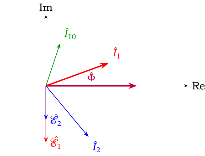
Рис. 17.14. Векторна діаграма трансформатора в режимі навантаження. Потік \hat{\Phi} напрямлений уздовж дійсної осі; ЕРС відстають від нього на \pi/2 ; струм \hat{I}_1 є сумою струму холостого ходу та скомпенсованого вторинного струму.
