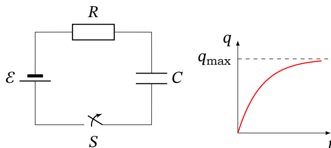
Рис. 7.17. Зарядка конденсатора від джерела ЕРС через резистор: коло та графік q(t)
