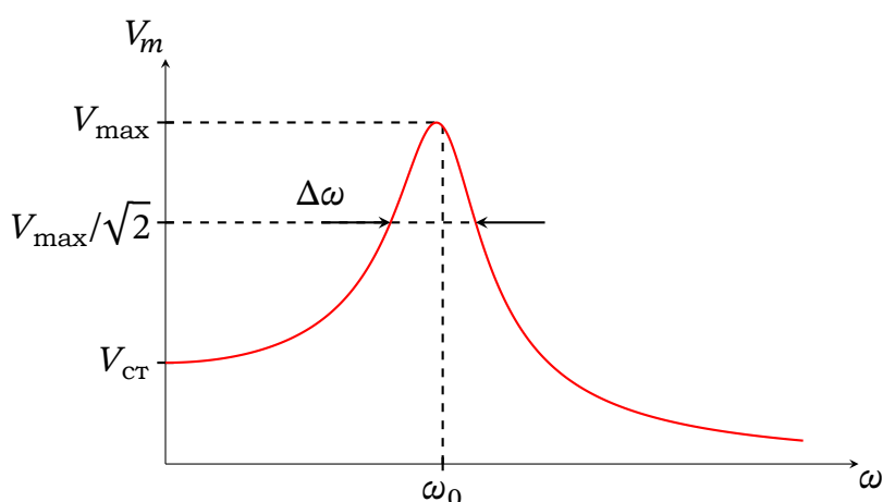
Рис. 17.7. Характеристики резонансної кривої: V_{\max} — максимум амплітуди, V_{\text{ст}} — статична амплітуда, \Delta\omega — ширина резонансу.
