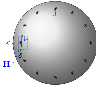
Рис. 13.10. Контур для оцінки циркуляції \mathbf{H} поблизу циліндричної поверхні провідника (вигляд зверху)
