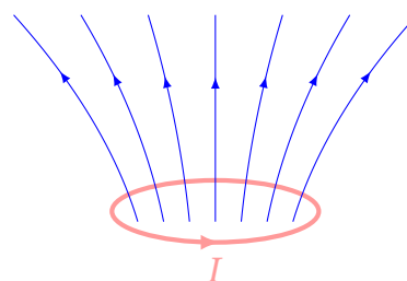
Рис. 11.9. Контур зі струмом I і створюване ним власне магнітне поле
