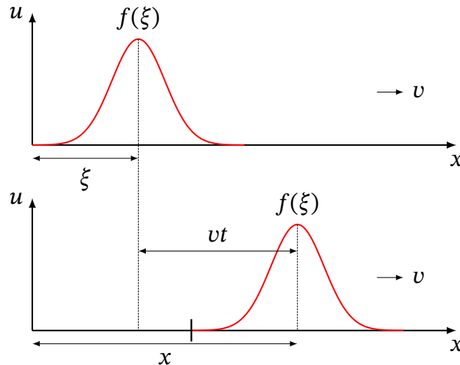
Рис. 15.2. Збурення, що поширюється без зміни форми зі швидкістю v : профіль у момент t — це профіль у момент 0, зсунутий на vt
