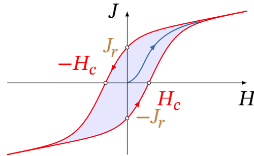
Рис. 11.12. Петля гістерезису феромагнетика: J_r — залишкова намагніченість, H_c — коерцитивна сила
