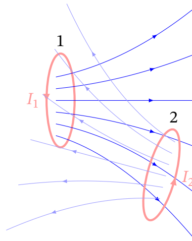
Рис. 12.14. Два нерухомих контури, магнітно пов'язані один з одним
