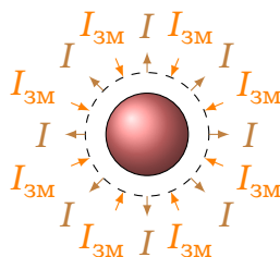
Рис. 13.3. Радіальне стікання заряду з кулі: струм провідності I і струм зміщення I_{\text{зм}}
