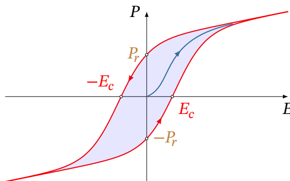
Рис. 7.3. Петля гістерезису сегнетоелектрика: P_r — залишкова поляризація, E_c — коерцитивна сила
