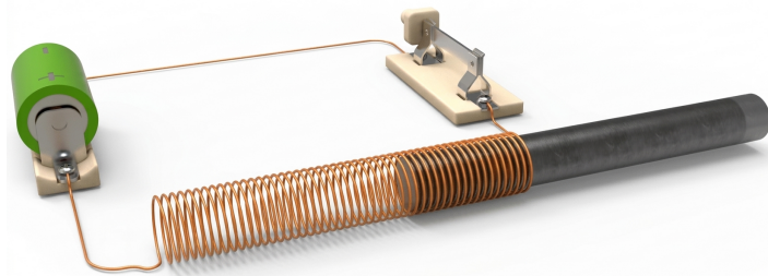
Рис. 12.19. Осердя втягується в котушку зі струмом — приклад пондеромоторної сили в магнітному полі
