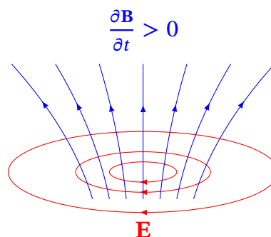
Рис. 12.9. Вихрове електричне поле, породжене зростаючим у часі магнітним полем
