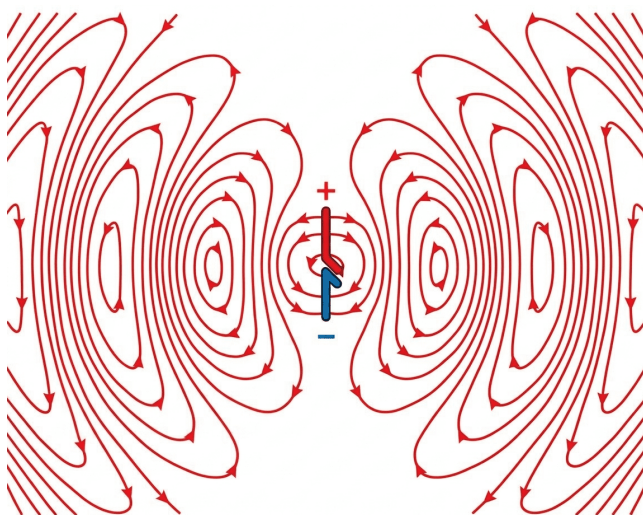
Рис. 15.7. Електричне поле осцилюючого диполя: у ближній зоні поле ніби «причеплене» до диполя, у хвильовій — випромінюється
