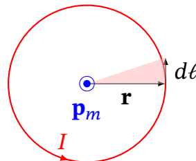
Рис. 10.12. До обчислення магнітного моменту колового витка зі струмом
