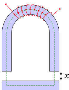
Рис. 12.20. Електромагніт з якорем, відокремленим повітряним зазором x
