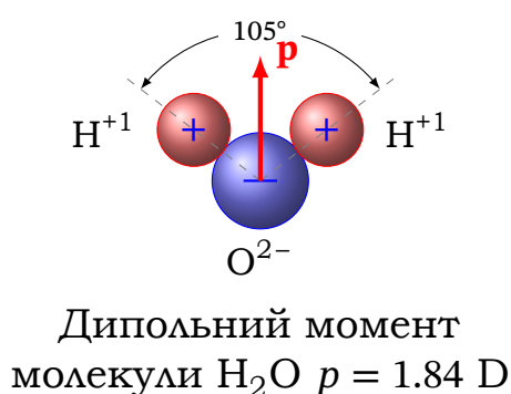
Рис. 3.2. Ілюстрація дипольних моментів деяких полярних молекул
