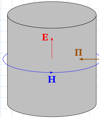
Рис. 12.9. Поля E , H і вектор Пойнтінга \Pi на поверхні довгого провідника зі струмом
