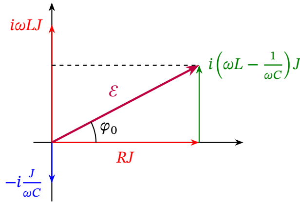
Рис. 16.7. Векторна діаграма для LCR -контурі, показаного на рис. 16.1, для випадку \omega L > 1/\omega C .
