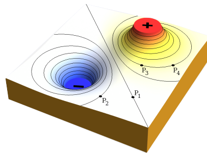
(б) Екіпотенціальні поверхні — карта висот в електростатичному полі!
