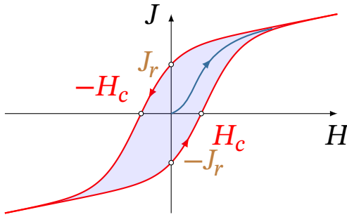
Рис. 9.11. Петля гістерезису феромагнетика: J_r — залишкова намагніченість, H_c — коерцитивна сила
