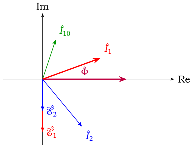
Рис. 18.14. Векторна діаграма трансформатора в режимі навантаження. Потік \Phi напрямлений уздовж дійсної осі; ЕРС відстають від нього на \pi/2 ; струм \hat{I}_1 є сумою струму холостого ходу та скомпенсованого вторинного струму.
