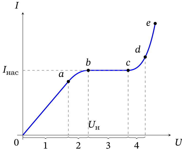
Рис. 8.7. Схематична вольт-амперна характеристика розряду в газі: омична ділянка (1), перехідна ділянка (2), струм насичення (3), лавинне зростання й пробій (4); точки a–e — характерні режими
