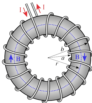
Рис. 11.11. Тороїдальна котушка
