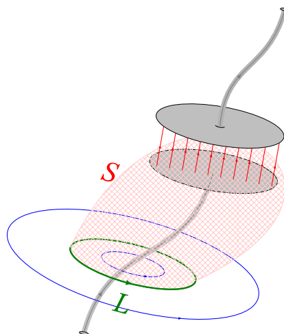
Рис. 12.2. Контур L , натягнута на нього поверхня S та провідник зі струмом, що її пронизує
