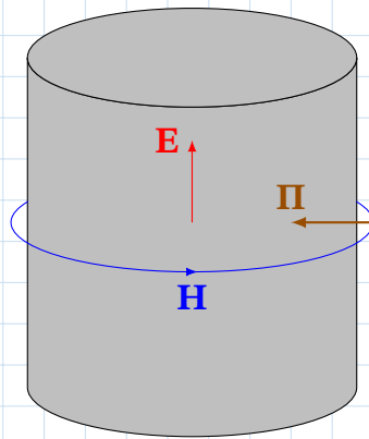
Рис. 12.9. Поля \mathbf{E} , \mathbf{H} і вектор Пойнтінга \mathbf{\Pi} на поверхні довгого провідника зі струмом
