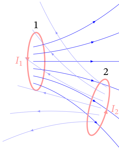
Рис. 11.14. Два нерухомих контури, магнітно пов'язані один з одним
