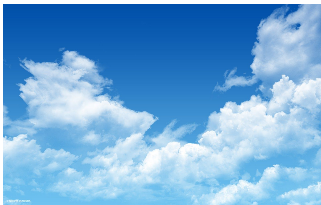
Рис. 15.10. Розсіювання сонячного світла молекулами атмосфери — причина блакитного кольору неба
