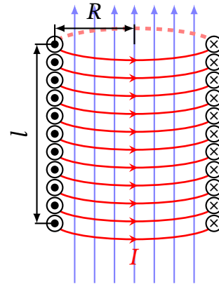
Рис. 11.18. Поздовжній переріз довгого соленоїда: однорідне поле всередині, струм у витках обмотки
