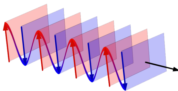
Рис. 14.3. Хвильовий вектор \mathbf{k} вказує напрям поширення плоскої хвилі й перпендикулярний до хвильових площин
