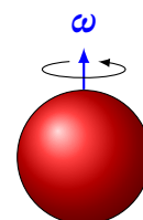
Рис. 8.13. Однорідно заряджена куля, що обертається навколо власної осі
