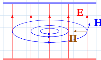
Рис. 12.8. Поля \mathbf{E} , \mathbf{H} і вектор Пойнтінга \mathbf{\Pi} при зарядці плоского конденсатора
