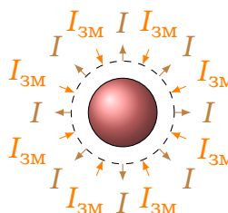
Рис. 12.3. Радіальне стікання заряду з кулі: струм провідності I і струм зміщення I_{\text{зм}}
