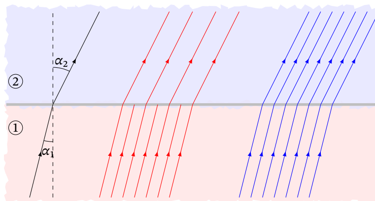
Поле вектора E Поле вектора D
