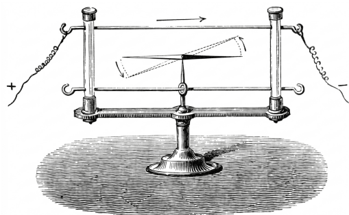
Рис. 9.1. Установка Ерстеда
